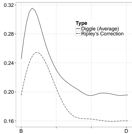
(d) \sqrt{\text{Var}(\hat{f})}, n = 1000
