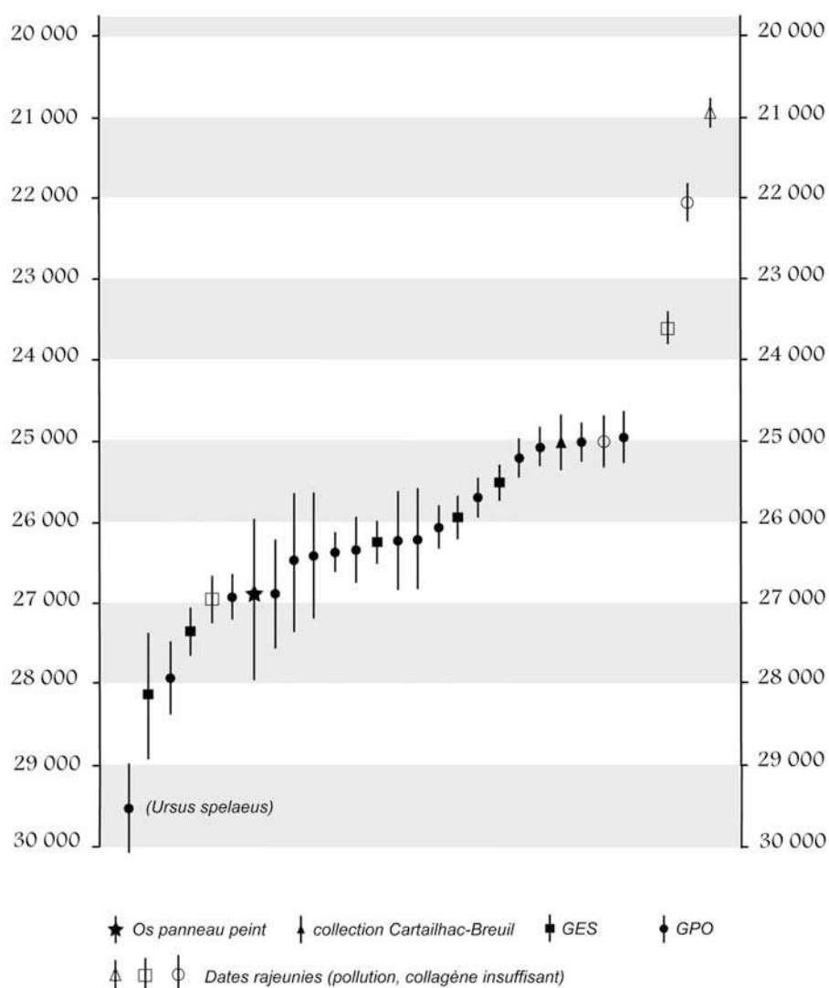
Fig. 5. Gargas, niveaux gravettiens (GES et GPO, et Cartailhac-Breuil) : dates ^{14}\text{C} (2 sigma) classées par ordre croissant.
