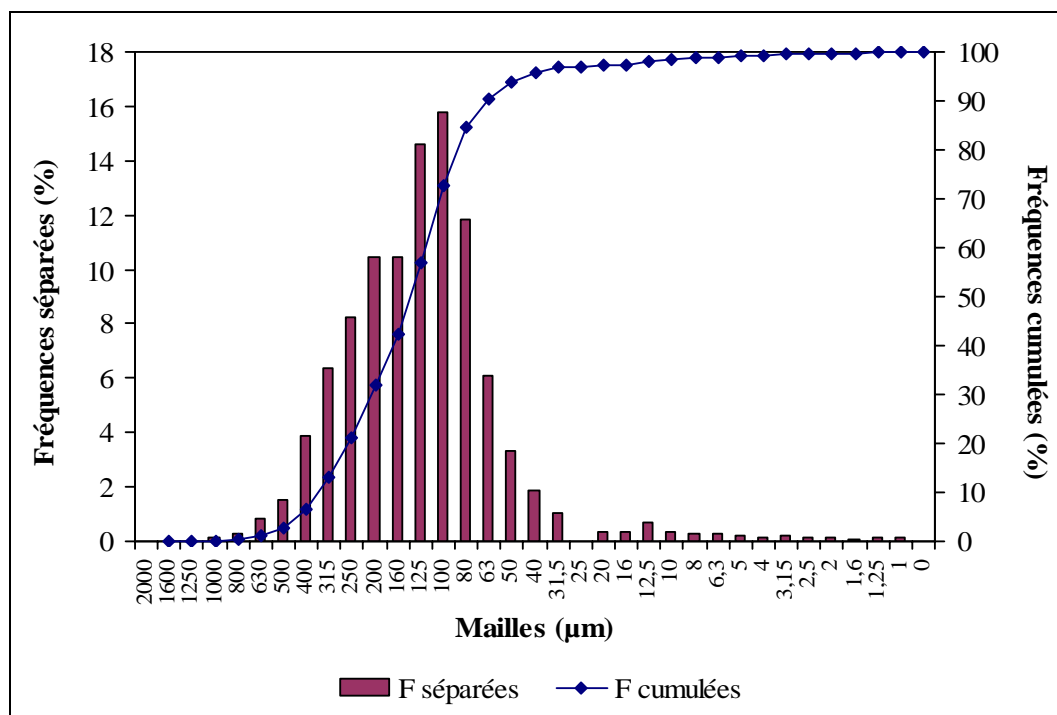
Figure 7 - Granulométrie de la terre fine de la très basse nappe alluviale post-romaine (Bordj La Gare).
