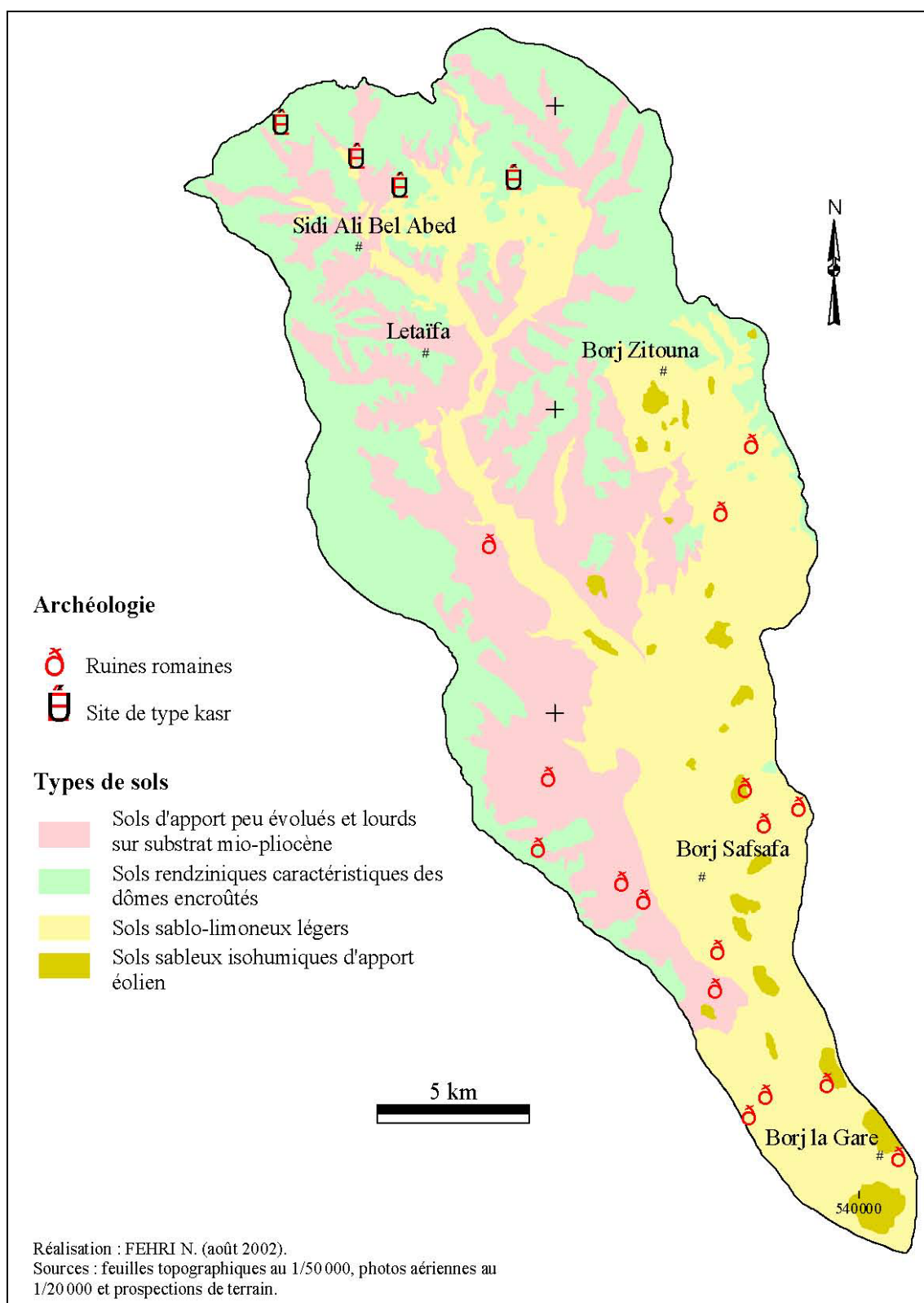
Figure 6 - Répartition spatiale des sites archéologiques en fonction des différents types de sols dans le bassin versant de l'oued Chaâl-Tarfaoui.
