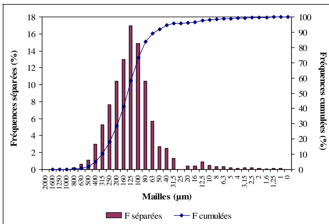
Figure 4 - Granulométrie de la terre fine de la basse nappe alluviale holocène pré-romaine (Bordj La Gare).
