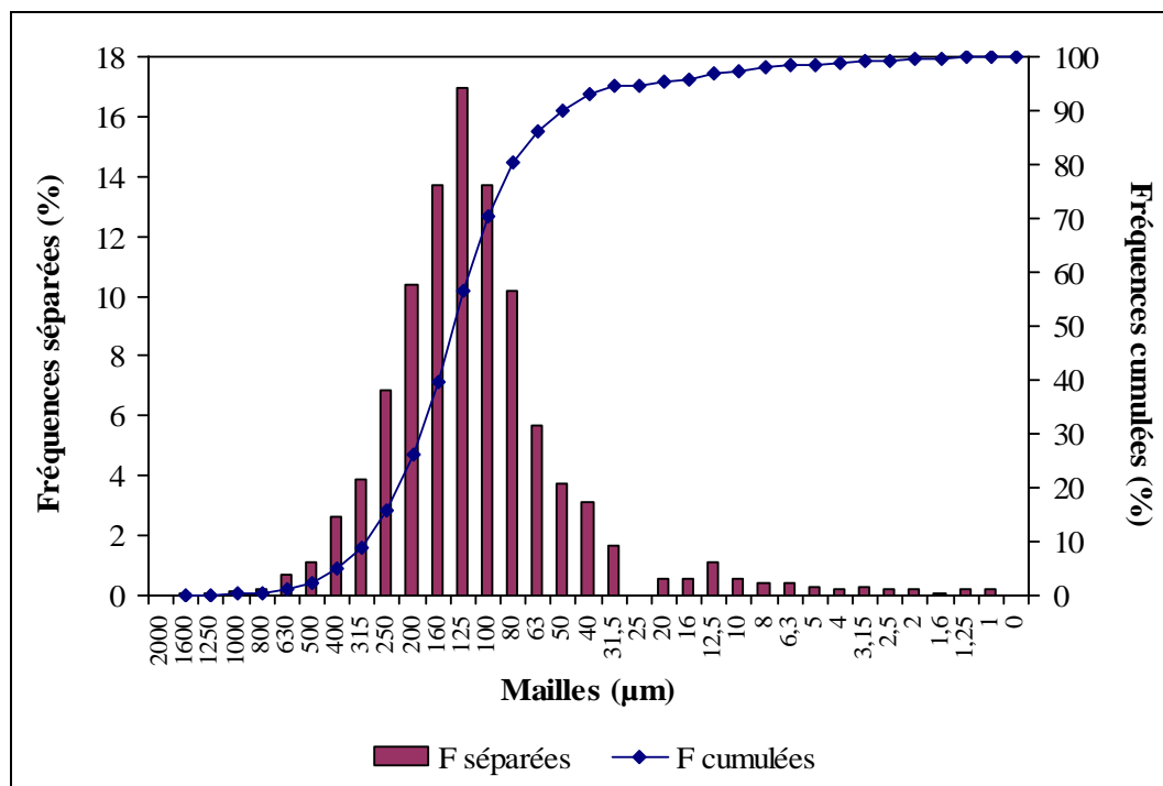
Figure 10 - Granulométrie de la terre fine des dépôts de la crue de 1969 à Borj La Gare (voir Fig. 2, niveau 3).
