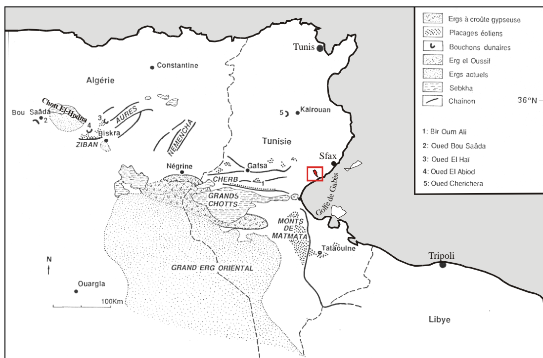
Figure 3 - Les accumulations de sables éoliens du Pléistocène supérieur entre les Ziban et le golfe de Gabès.
