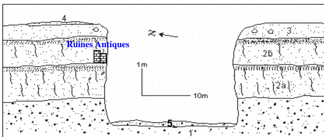
Figure 2 - Coupe de Borj La Gare sur l'oued Tarfaoui.
