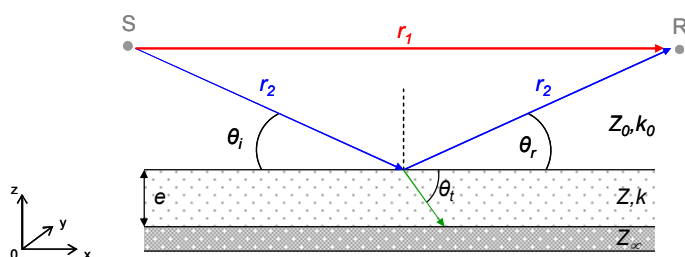
Figure 23. Représentation schématique de la configuration géométrique étudiée : Trajets des ondes directe ( r_1 en rouge) et réfléchie ( r_2 en bleu) de la source au récepteur, au-dessus d'un sol parfaitement plan et partiellement réfléchissant (matériau bicouche)
