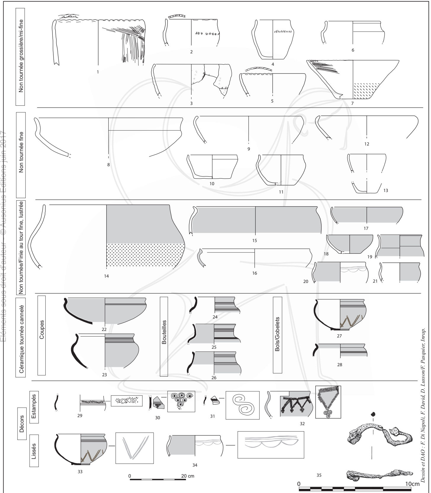
Fig. 3. Sublaines "Le Grand Ormeau" planche synthétique du mobilier de la phase 2, La Tène A2-La Tène B1 (425-350 a.C.) (échelle 1/8 e pour la céramique, 1/2 pour le mobilier métallique ; dessin et DAO F. Di Napoli, F. David, F. Pasquier et D. Lusson, Inrap).
