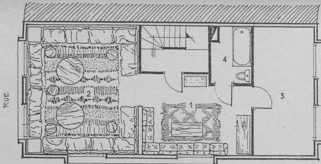
2 e ETAGE
