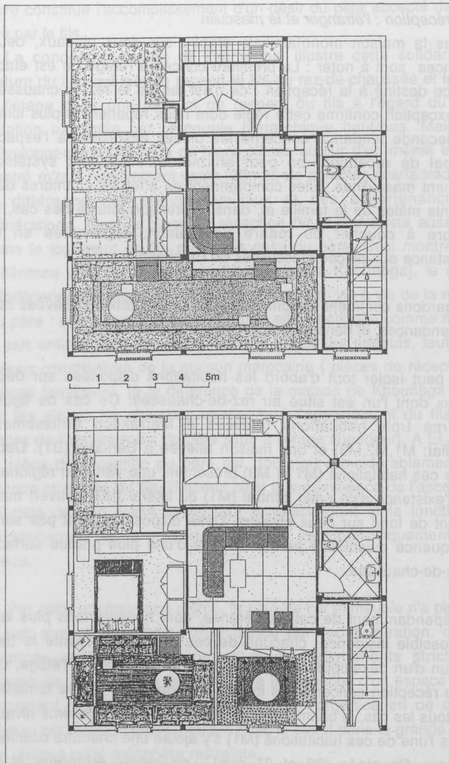
Fig .26 Plans d'une maison dont le rez-de chaussée est habité par le fils aîné et l'étage par le père (El jadida, relevé EJ3, dessin Jaâfar BOULEJIOUCH).
