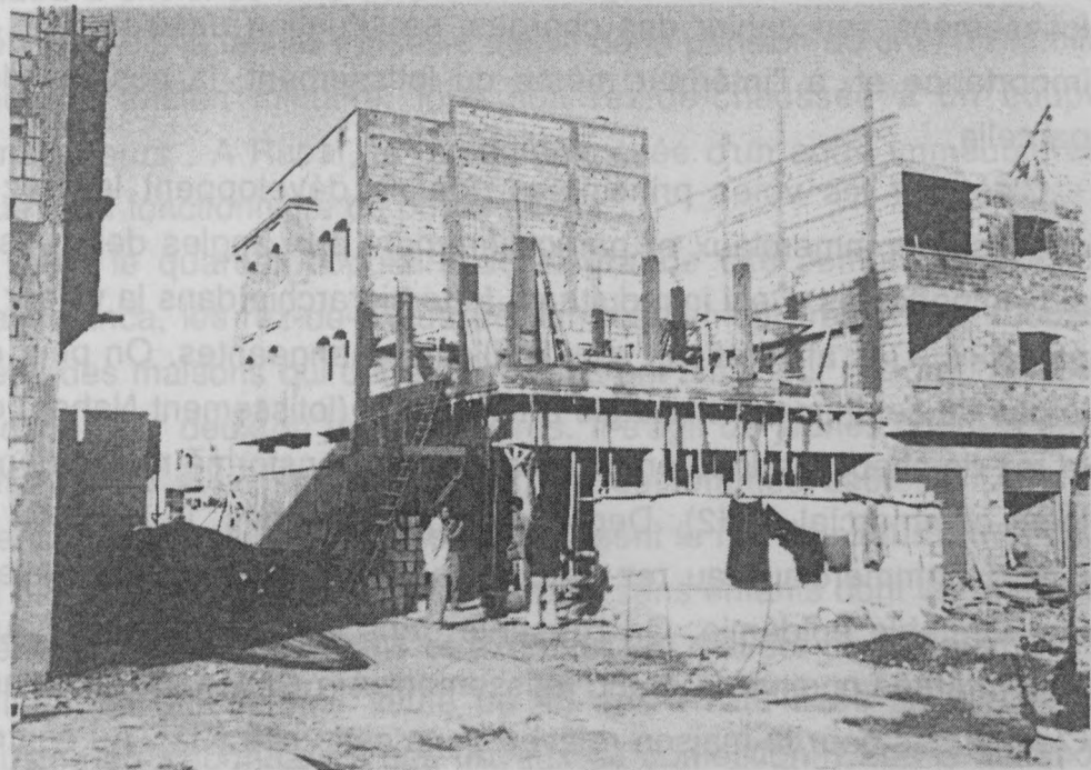
PL.10 La construction des maisons dans le lotissement Aïn Chock: deux moments de la mise en oeuvre du système poteau-dalle.
