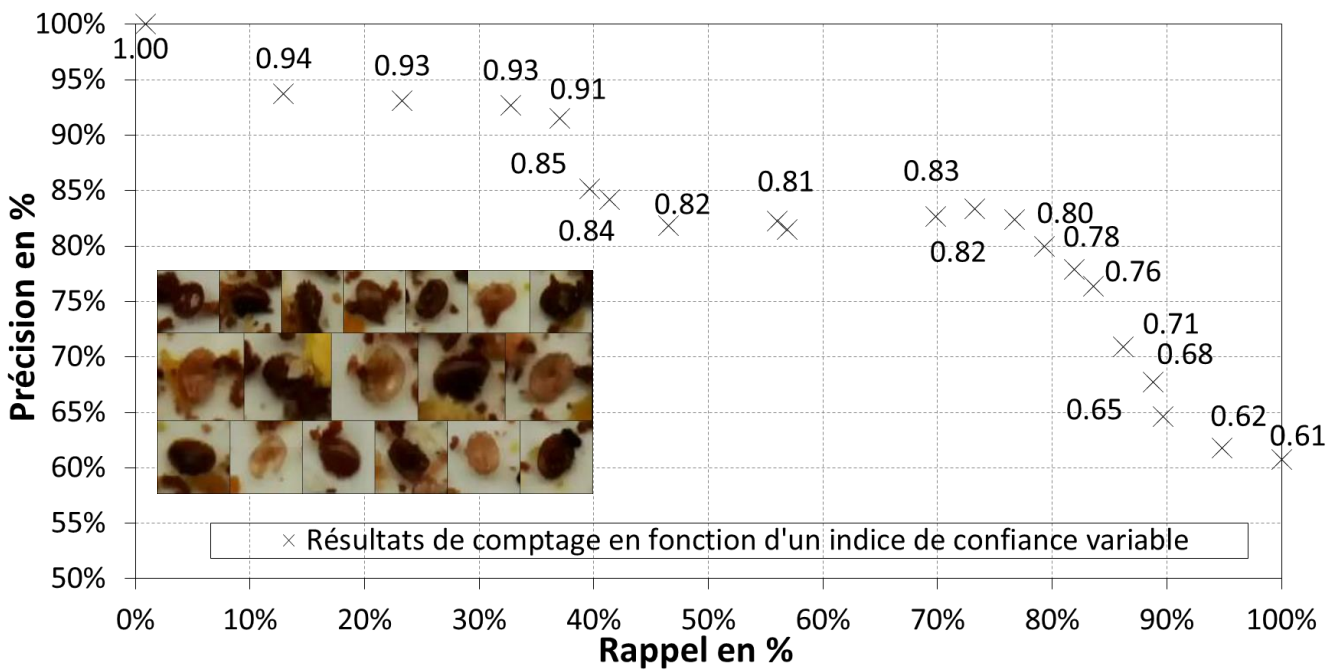
Graphique de précision, rappel et mosaïque des varroas détectés sur un lange
