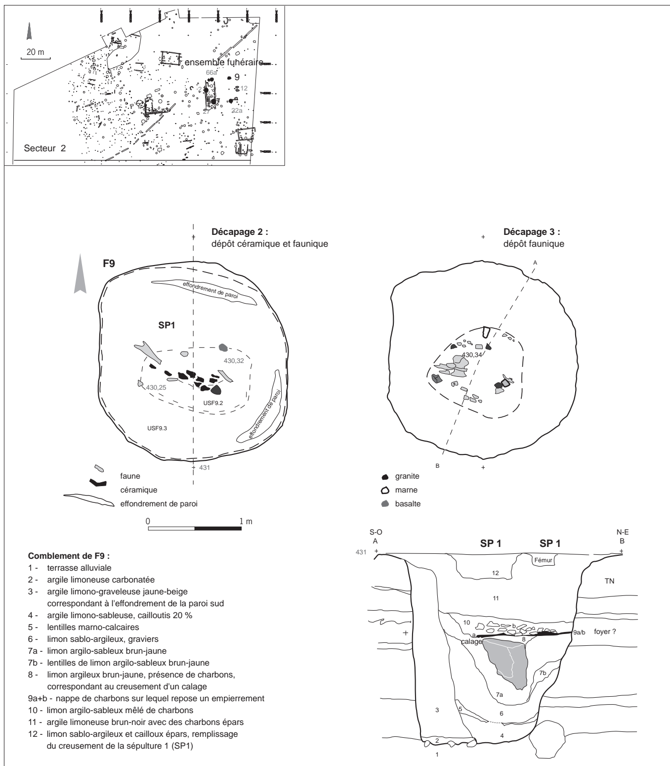
Fig. 98 : Artière-Ronzière. Relevés et vues en plan et en coupe de la fosse F9 (relevés et cliché S. Saintot).
