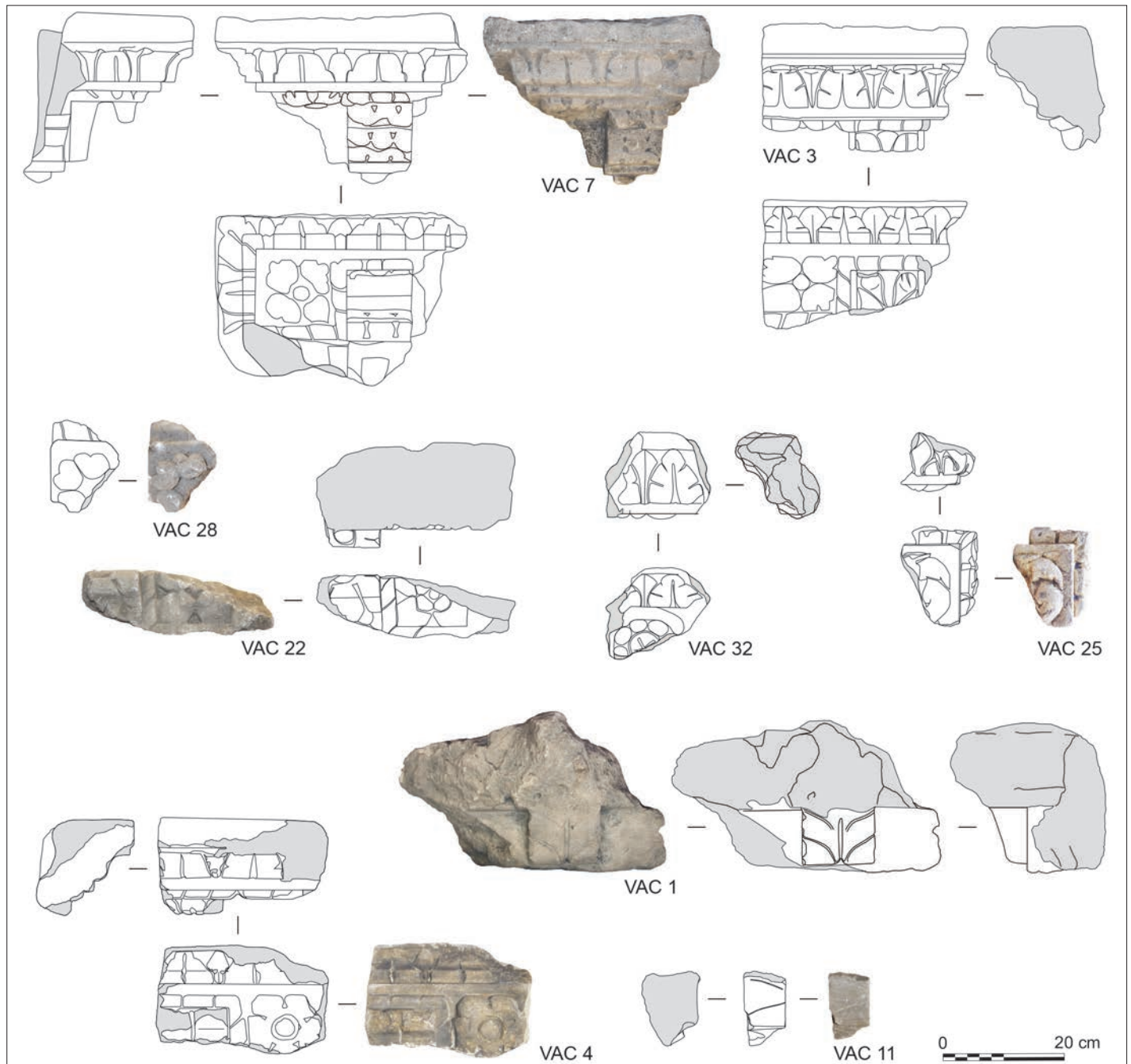
Fig. 10 – La corniche modillonnaire corinthienne et ses variantes décoratives (DAO et clichés : D. Mattiuz).
