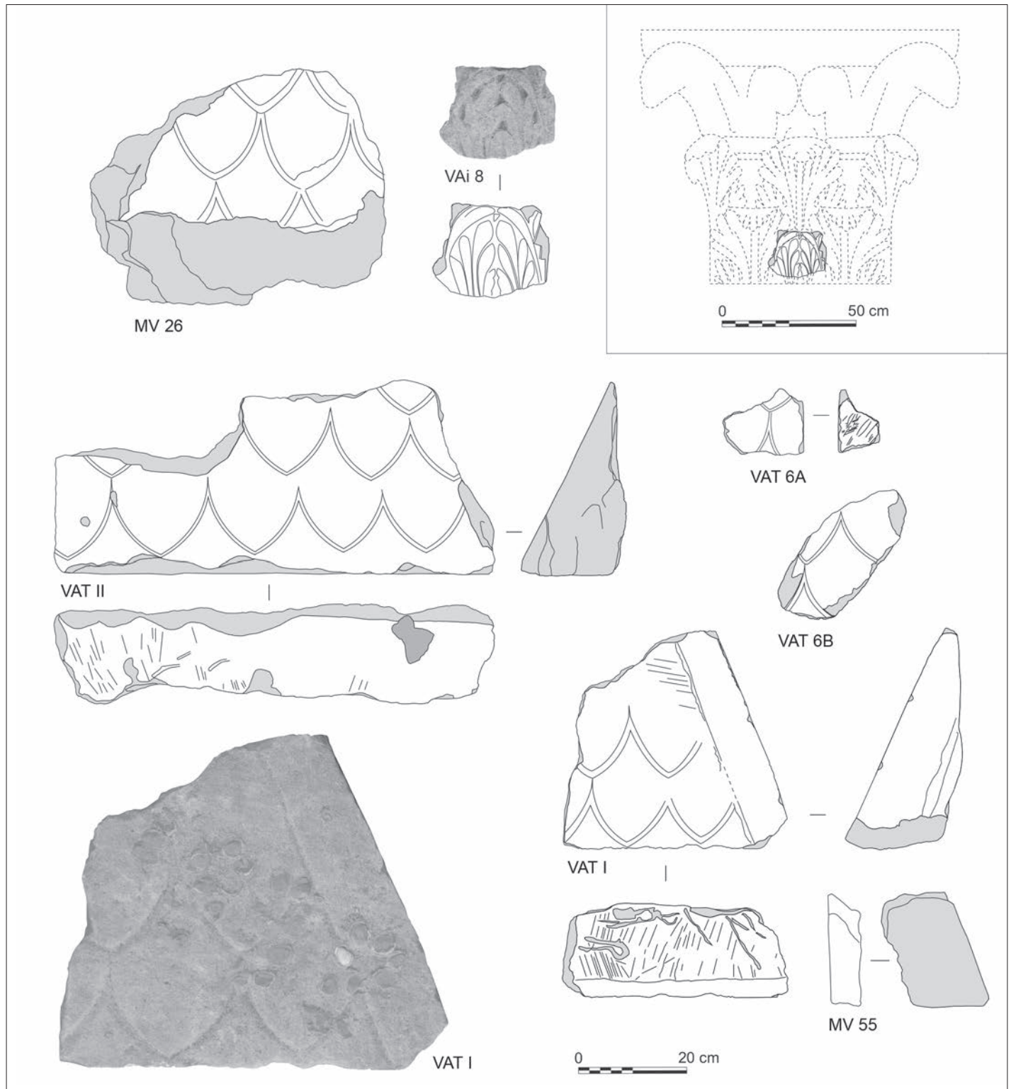
Fig. 13 – Blocs de couverture et chapiteau sommital (DAO et clichés : D. Mattiuz).
