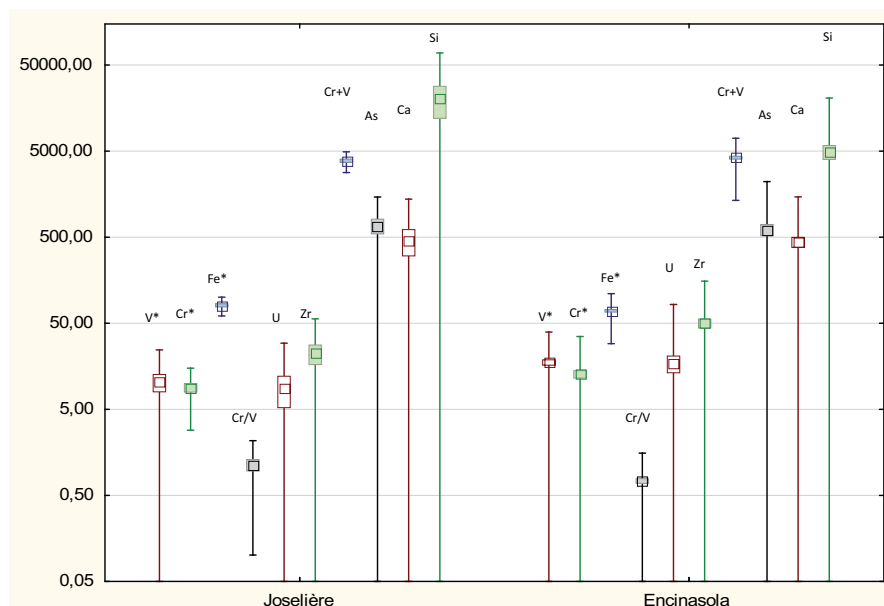
Fig. 6 : Comparaison des compositions chimiques des objets en variscite du site de la Joselière (44) avec celles du gisement d'Encinasola. Même légende que fig. 4.
