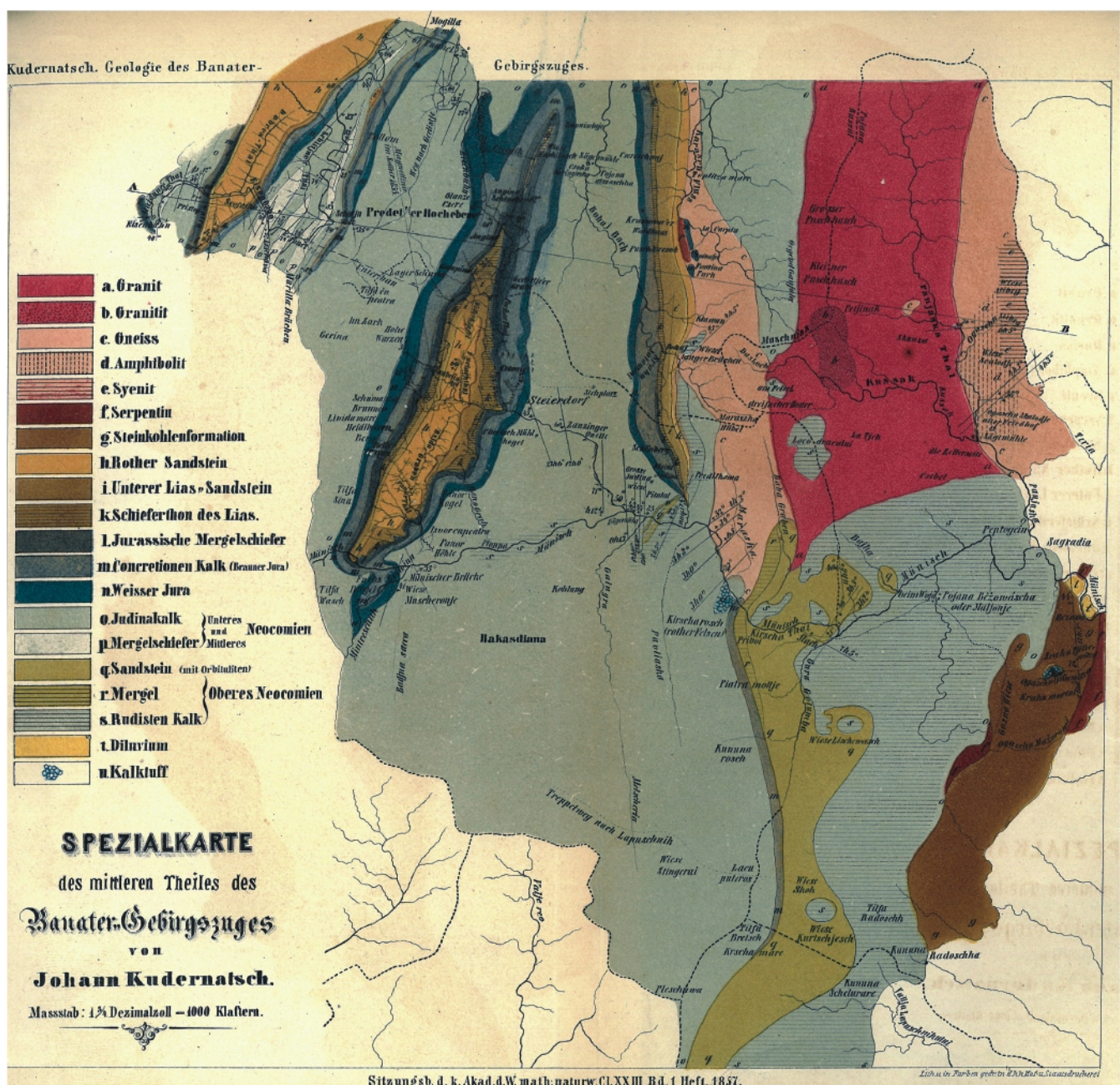
Figure 2: Spezialkarte des mittleren Theiles des Banater Gebirgszuges (Kudernatsch, 1857a). Source: Library of the Geological Survey of Austria.
