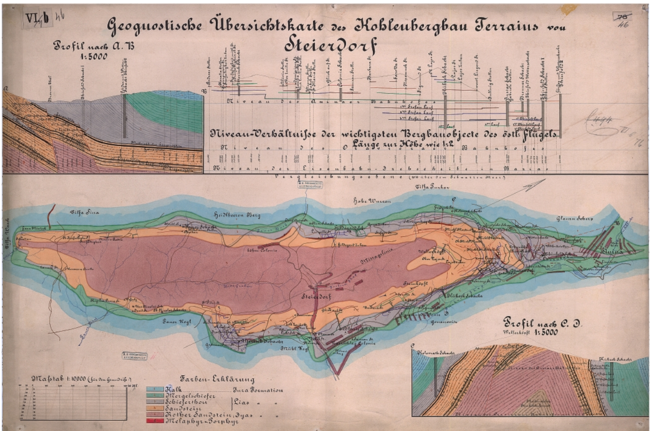
Figure 5: Geognostische Übersichtskarte des Kohlenbergbau Terrains von Steierdorf (***, 1872[?]). Source: Library of the Geological Survey of Austria.
