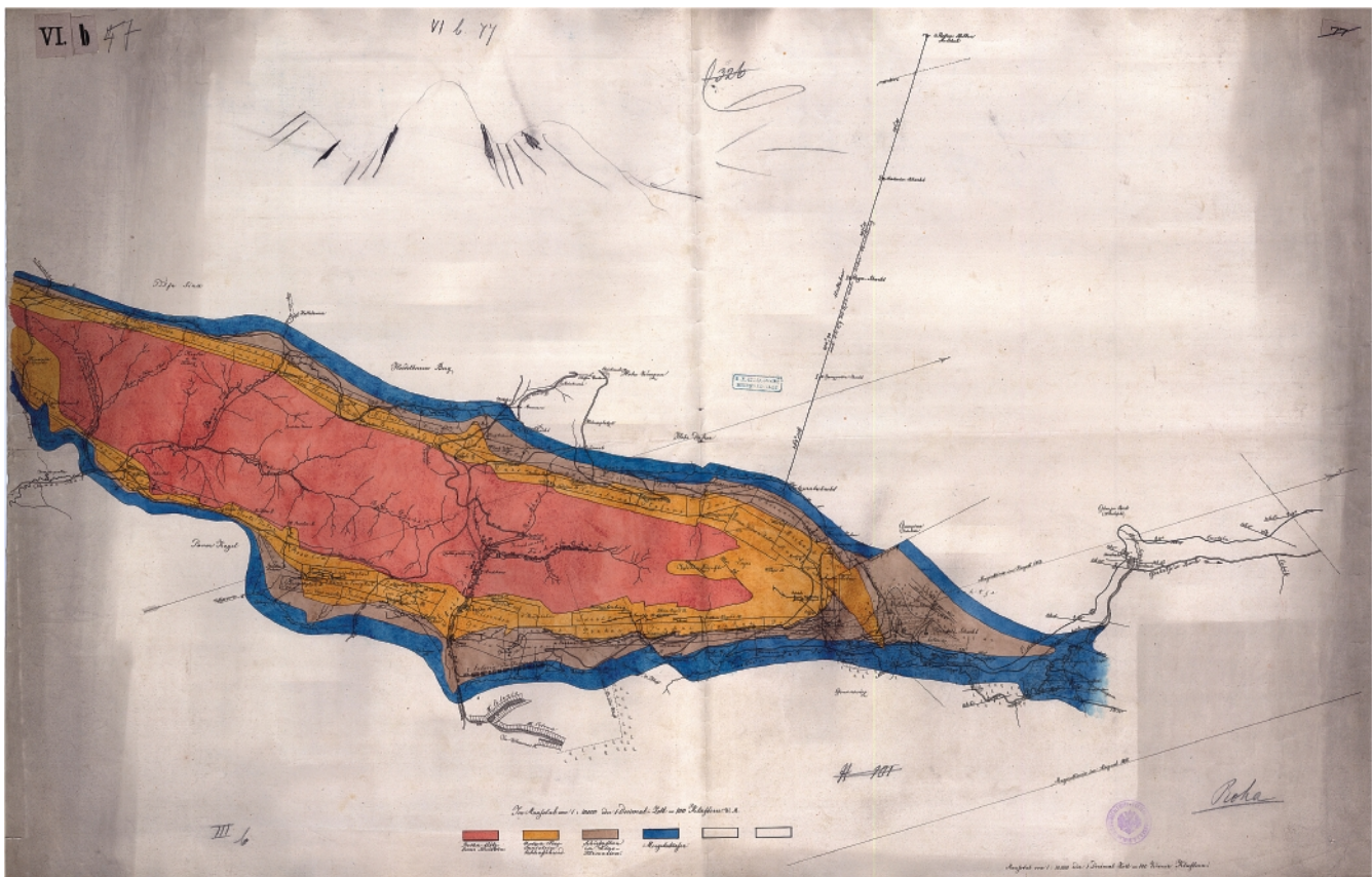
Figure 4: Geologische Karte von Steierdorf im Banat (Roha, 1867a[?]). Source: Library of the Geological Survey of Austria.
