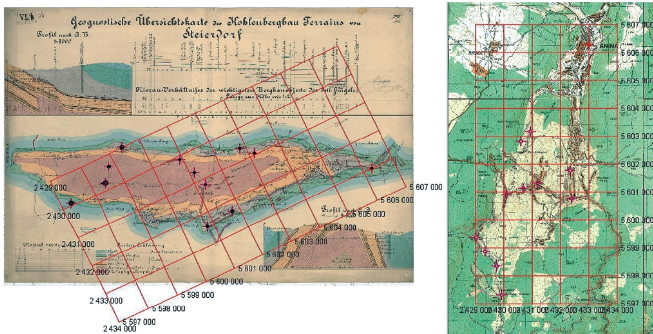
Figure 10: Analysis of the map Geognostische Übersichtskarte des Kohlenbergbau Terrains von Steierdorf (***, 1872[?]) visualised in MapAnalyst.
