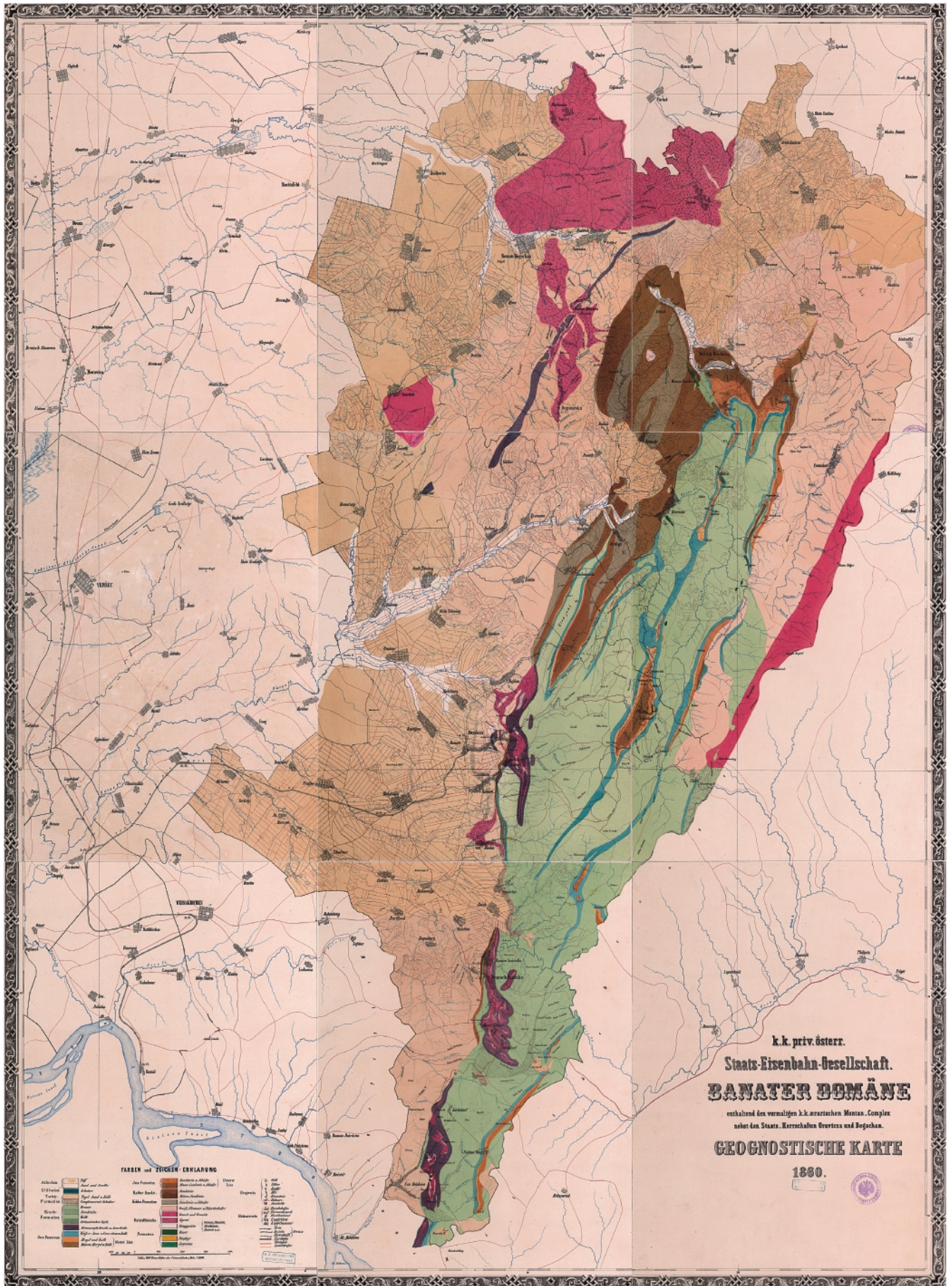
Figure 3: Banater Domäne: enthaltend den vormaligen k. k. aerarischen Montan-Complex nebst den Staats. Herrschaften Oravicza und Bokschan: Geognostische Karte (***) [Foetterle], 1860). Source: Library of the Geological Survey of Austria.
