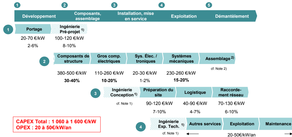
Figure 6 Chaîne de valeur dans le secteur éolien
