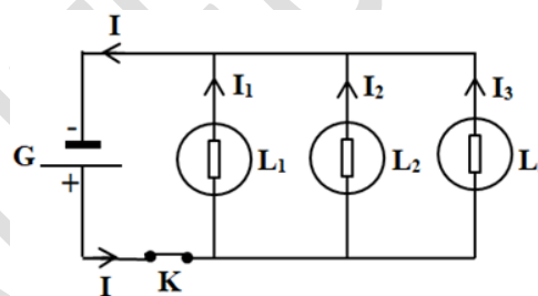
(b) : Schéma du circuit électrique en parallèle
