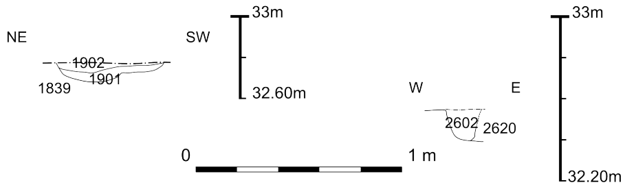
Qalhât 2013 B94.D ST138 Coupe WE et plan
