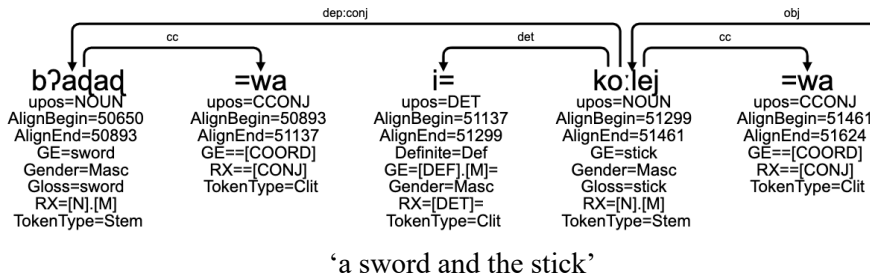
Figure 15. Nominal coordination (UD-style)
