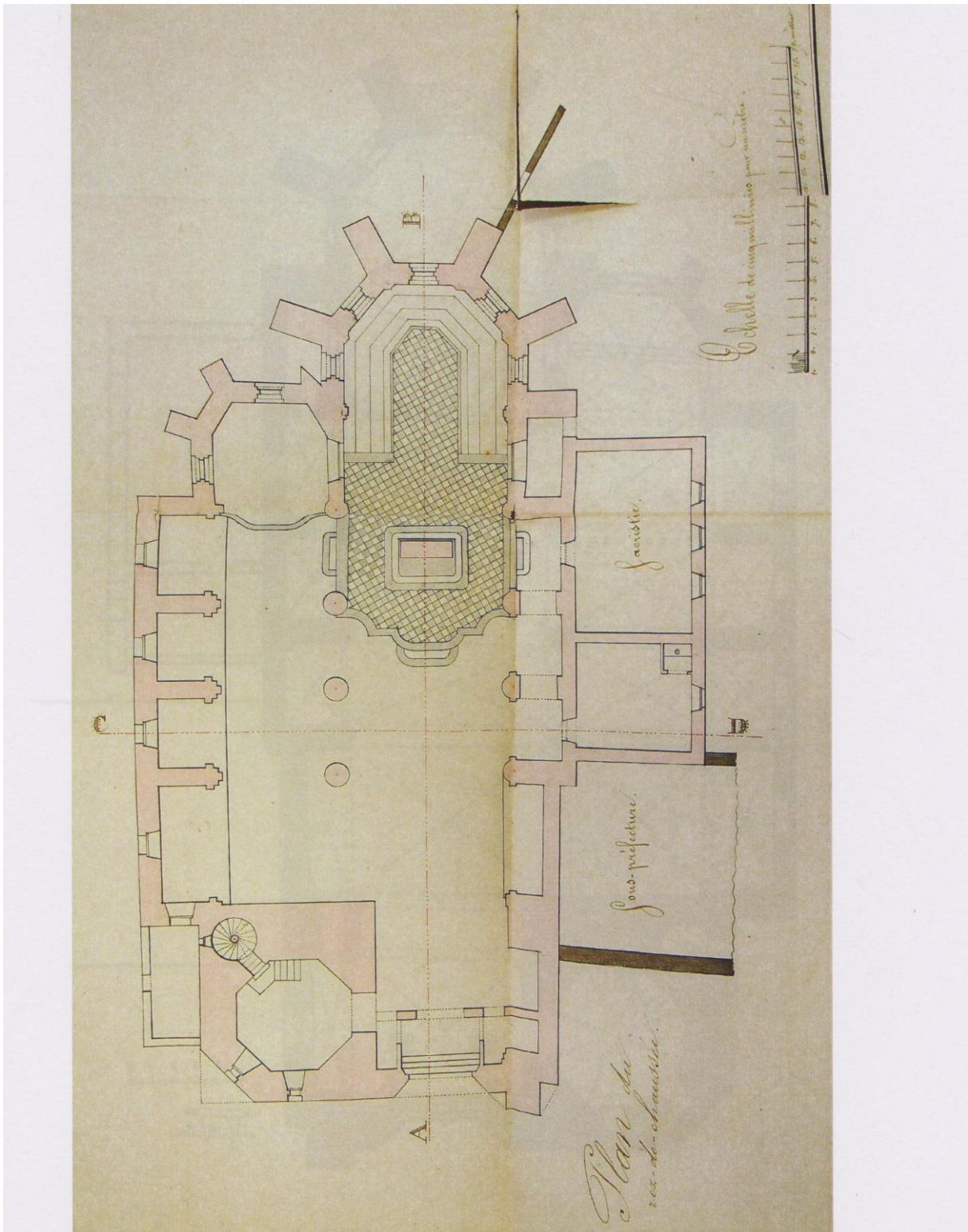
Fig. 2 : Lombez, ancienne cathédrale Sainte-Marie, plan au sol de 1841 levé par l'agent Voyer (extrait de Noémie OLLIER, Une abbatale élevée au rang de cathédrale au début du XIV e siècle : le cas de Notre-Dame de Lombez (XII e -XVIII e siècle) , mémoire de Master 2, Université de Toulouse-Le Mirail, 2013, vol. 2, p. 16).
