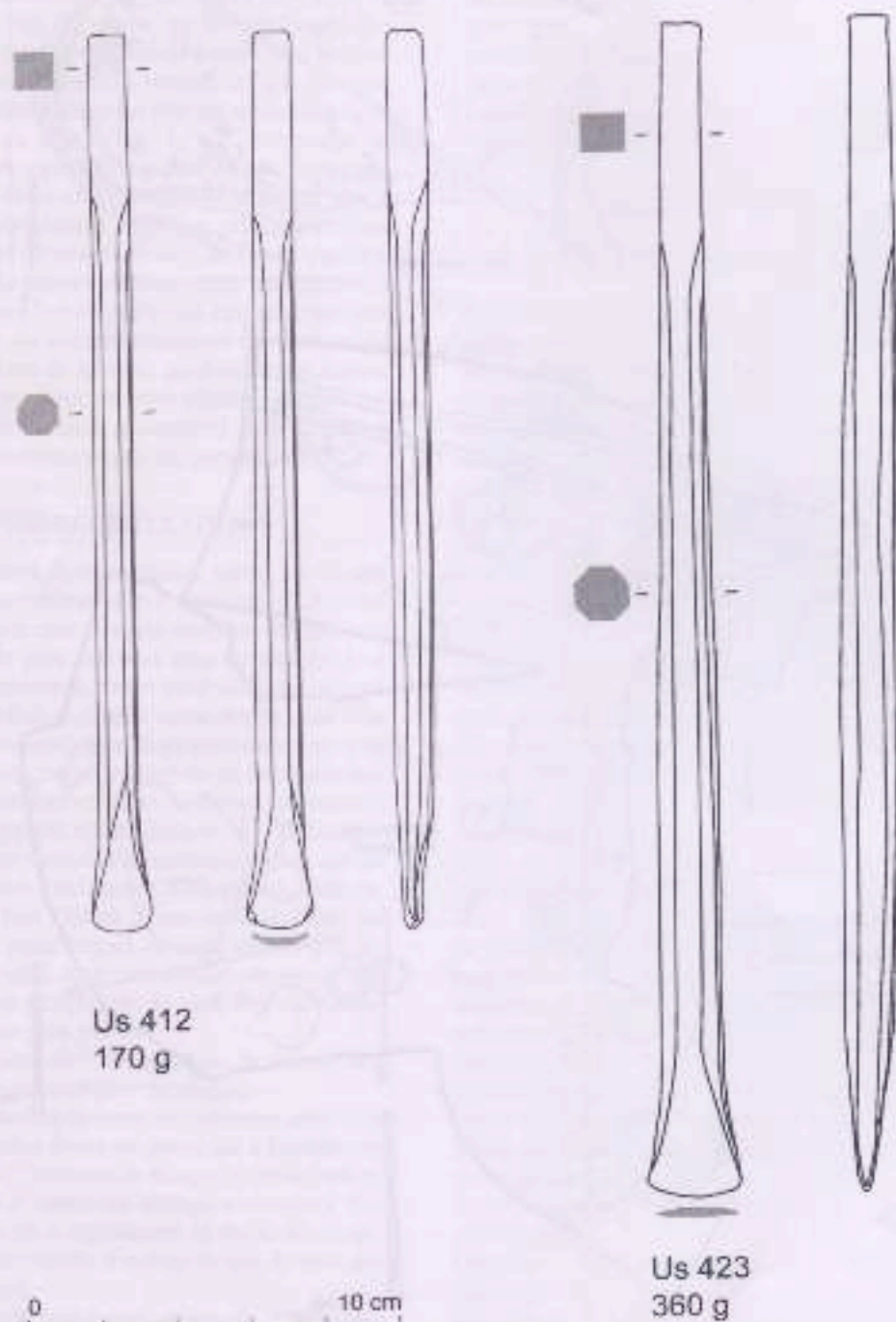
Fig. 2 - Les deux outils en alliage cuivreux découverts. À gauche, la gouge-burin (us 412), à droite, le grand ciseau (us 423). Dessins M. Michler. Fig. 2 - The two bronze tools. On the left: the gouge-burin (us 412), on the right the big graver (us 423). Drawings M. Michler.
