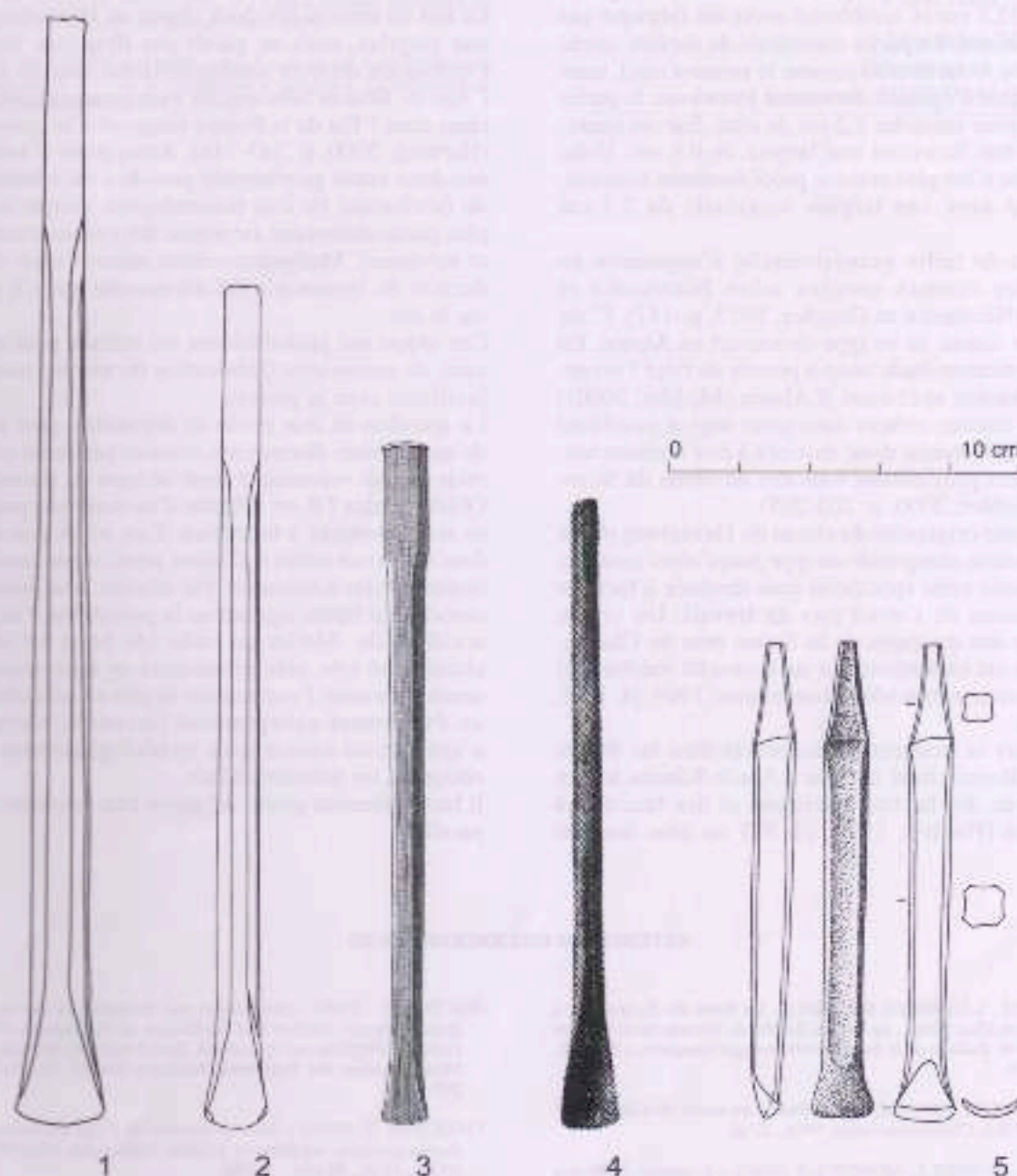
Fig. 3 – Planche comparative. N° 1 et 2 : gouge et ciseau provenant du Hexenberg ; n° 3 : ciseau provenant de Peschiera (d'après Montelius, 1895) ; n° 4 : gouge provenant de Zurich-Haumesser (d'après Wyss, 1971) ; n° 5 : gouge provenant du dépôt de Brno-Liesen (d'après Rihovsky, 1992).
