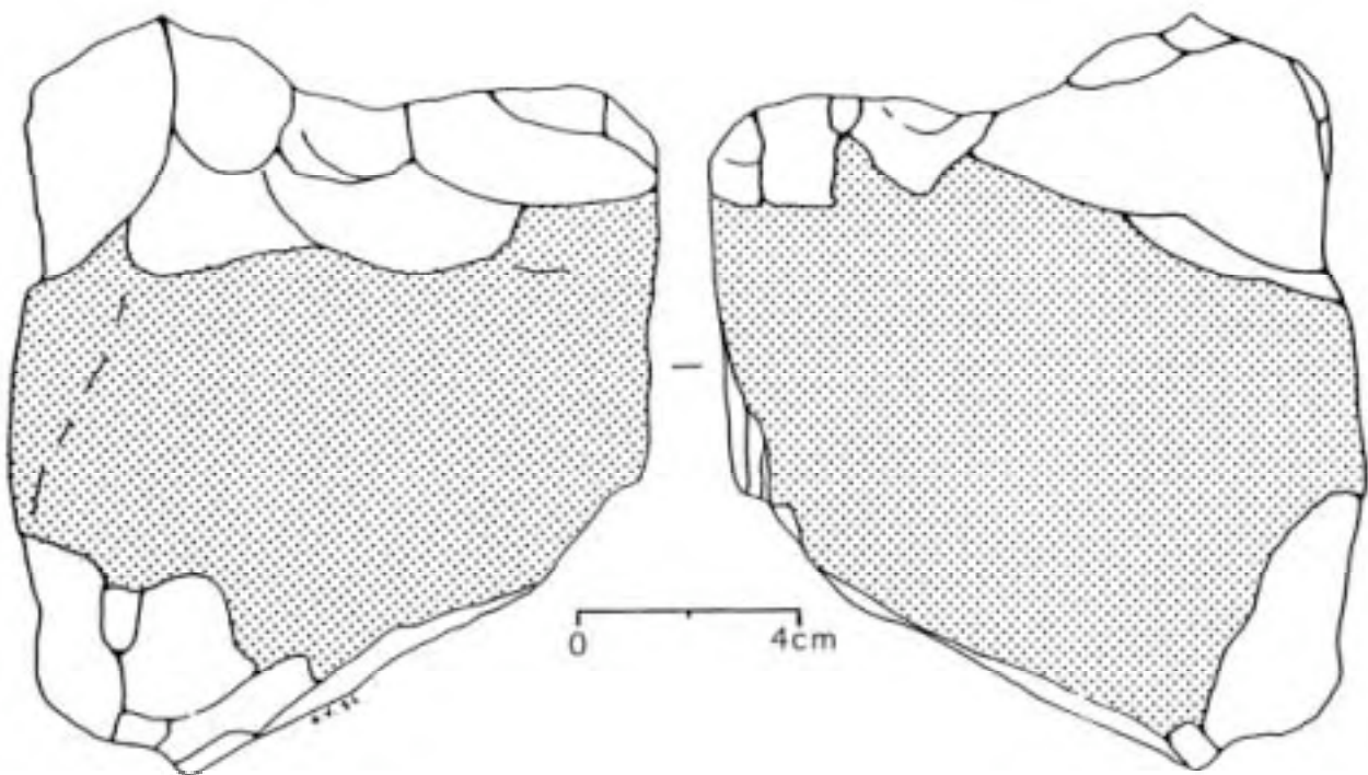
Figure 3 : téphrofact de la troisième nappe de recouvrement pyroclatique issue du Puy Chopine (récolte et dessin G. Vernet).
