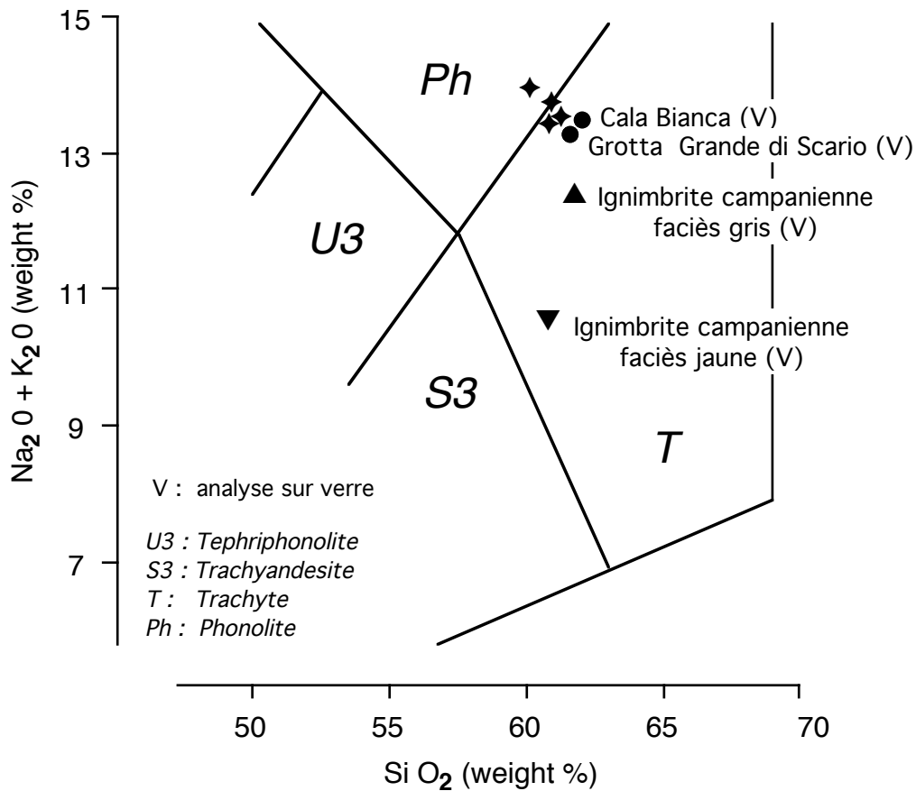
Figure 2 - Téphras identifiées entre Camerota et Scario et analyses de références pour l'ignimbrite campanienne (Barberi et al. , 1978) dans le diagramme SiO 2 /Na 2 O+K 2 O de Le Bas et al. (1986). Chemical composition of tephras identified between Camerota and Scario and reference analysis for the Campanian Tuff (Barberi et al. , 1978) in SiO 2 /Na 2 O+K 2 O diagram (Le Bas et al. , 1986).
