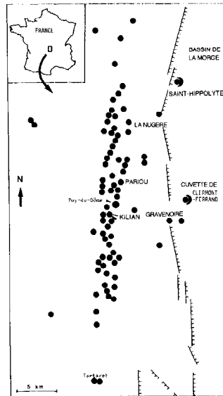
Fig. 1 - Carte schématisée de la Chaîne des Puys (d'après Camus et al. , 1983). Les volcans sont représentés par des points noirs. Zone d'étude en hachures et mention des principales localités étudiées.
