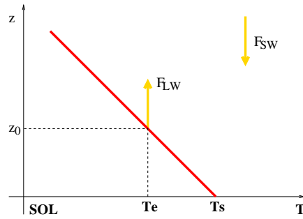
FIG. 1.1: Schéma de l'effet de serre : l'altitude équivalente d'émission est z_0 , à une température T_e . Le flux solaire entrant F_{SW} est égal au flux sortant F_{LW} . Le système est à l'équilibre.
