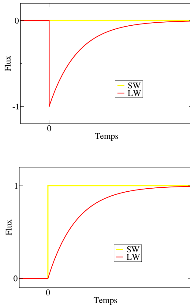
FIG. 3.1: Représentation schématique des deux expériences : GES en haut, où le flux LW est perturbé; SW en bas, où le flux SW est perturbé. Dans les deux cas, l'aire entre les deux courbes donne la quantité d'énergie supplémentaire stockée par la planète terre suite à la perturbation.
