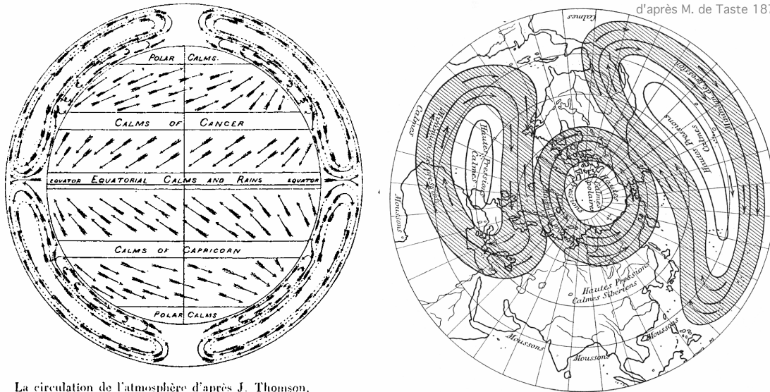
La circulation de l'atmosphère d'après J. Thomson.
