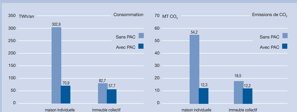
Figure 37 : Consommations et émissions de CO 2 globales selon une simulation statique établie sur le parc de logements existant en 2000
