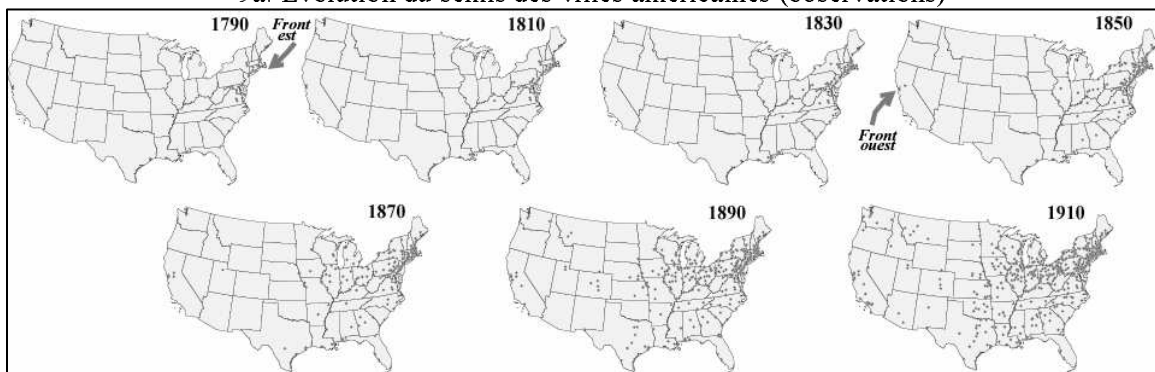
Figure 9 : Un mécanisme de front pionnier dans un pays neuf
