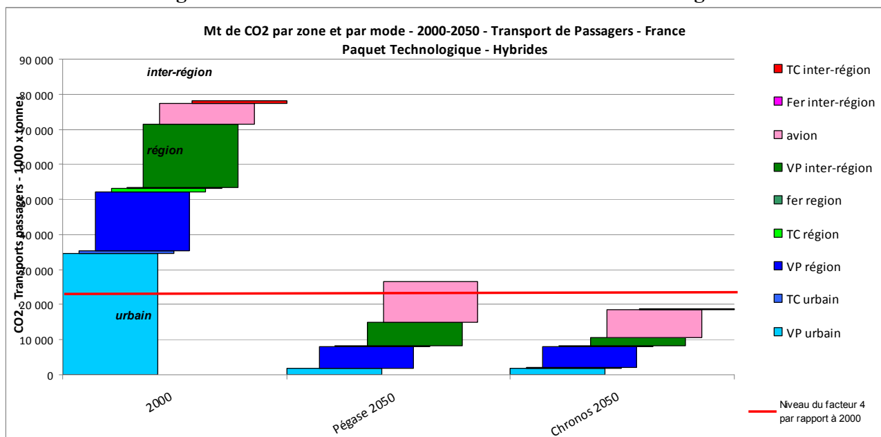
Figure 7 Emissions GES en 2050 scénario Chronos-Passagers
