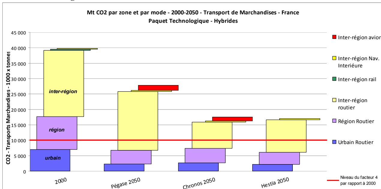
Figure 11 Emissions GES en 2050 scénario Hestia-marchandises
