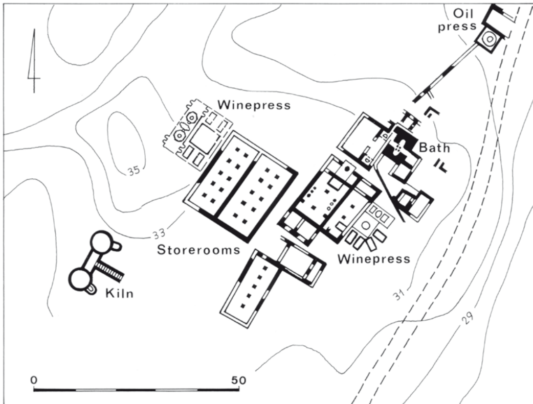
Fig. 11. Four à chambre double spécialisé dans la production de LRA 4B (VIe s.) associé à deux grands pressoirs à vin (Israel 1993a).
