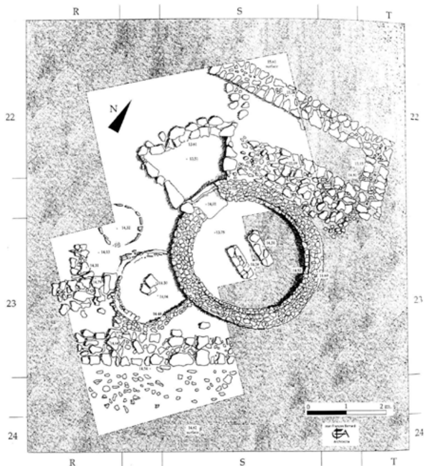
Fig. 7. Plan du four 2 ayant produit au VI e s. des amphores à pâte calcaires (Kassab Tezgör et Tatlican 1998, Fig. 11).
