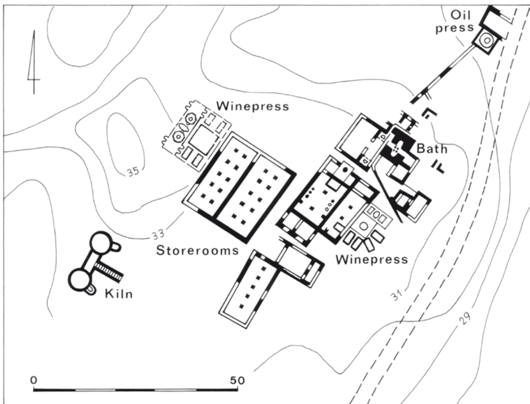
Fig. 11. Four à chambre double spécialisé dans la production de LRA 4B (VIe s.) associé à deux grands pressoirs à vin (Israel 1993a).
