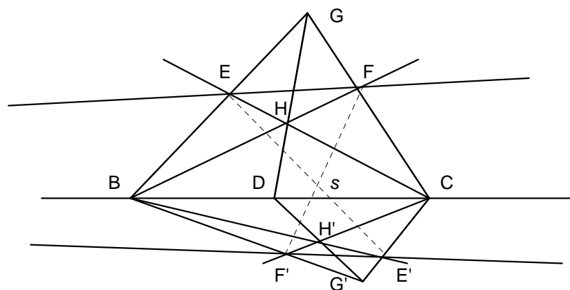
Figure 4 : le point S désigne le sommet du cône à quatre arêtes dont les deux quadrilatères EGFH , E'G'F'H' sont les sections. Par rapport à la figure 2, le point A a disparu : il est hors de l’espace limité donné, et donc de la figure.
