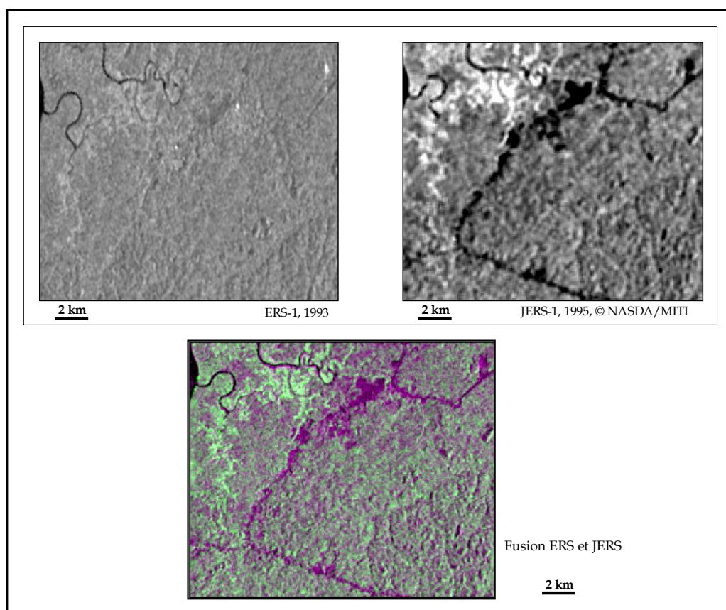
Figure 7. Fusion d'images radar pour améliorer la visu-interprétation de l'occupation du sol à Charvein
