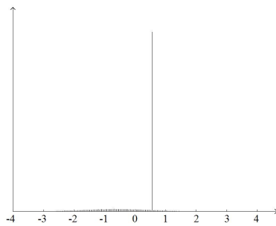
(F.b) \Delta(0, 1, -\frac{2}{\sqrt{3}}, \frac{10}{9})
