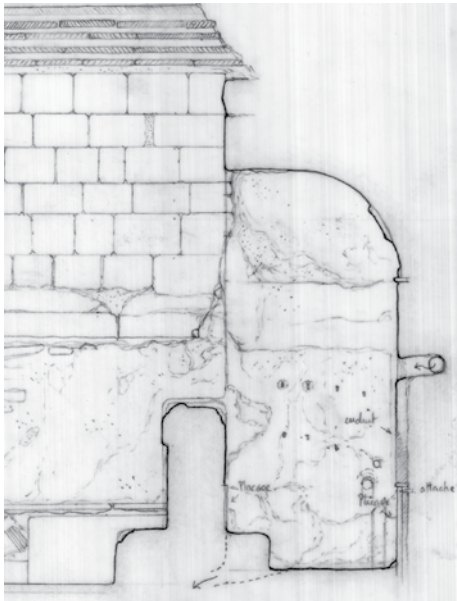
Fig. 6 Minute de relevé de la coupe est-ouest sur la baignoire de la salle 4.
