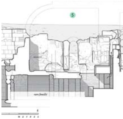
Fig. 14 (Ci-contre) vue vers le nord. Dans les hypocaustes, vue depuis le massif arc vers la salle (5) et les pillettes circulaires portant les bipédales.
