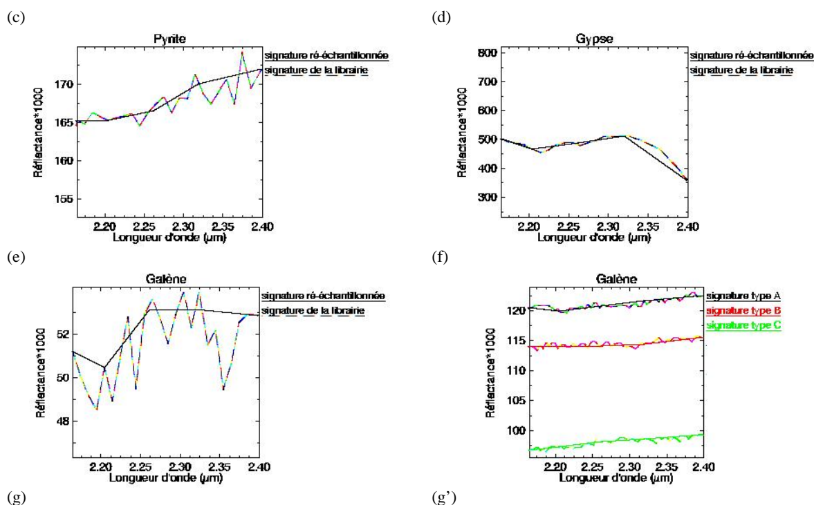
Figure 9 : Spectre de réflectance original de la librairie USGS et ré-échantillonné de la goethite (a), l'hématite (b), la barytine (c), la sphalérite (d), la pyrite (e), le gypse (f) et la galène (g), et (g') de la librairie JPL.
