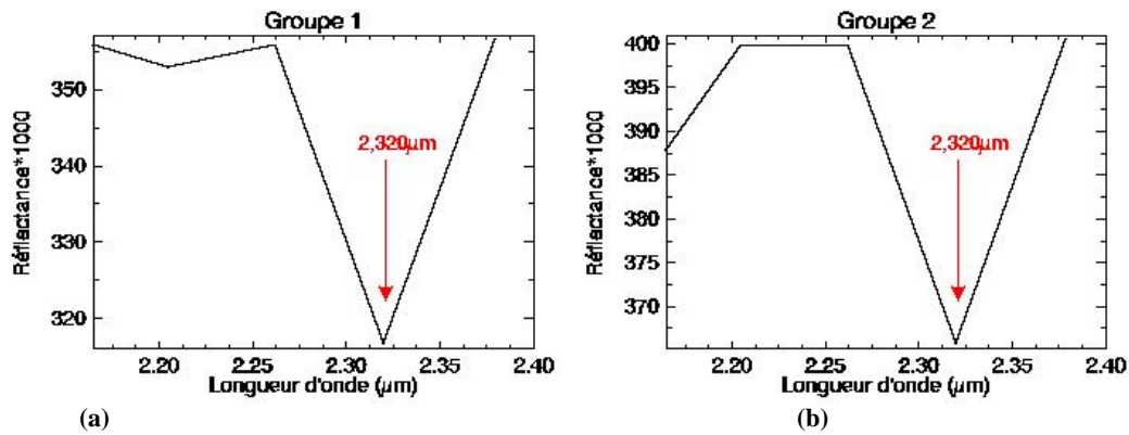
Figure 4 : Les signatures spectrales des rejets miniers (a) et (b) dans le domaine SWIR d'ASTER Figure 4: ASTER SWIR mine tailing spectral reflectance (a) and (b).
