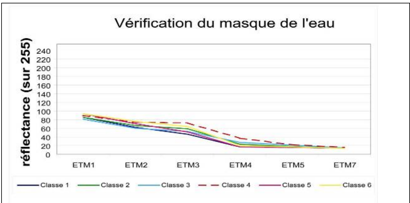
Figure 9, courbes radiométriques du masque de l'eau. On observe que la courbe radiométrique de la classe 4 présente une pente faible entre TM3 et TM4 avec des valeurs assez fortes de luminance sur TM3, 4 et 5. Il s'agit certainement de tannes légèrement inondés et non de surfaces en eau.
