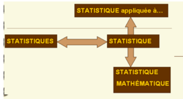
Figure 4 Statistique
