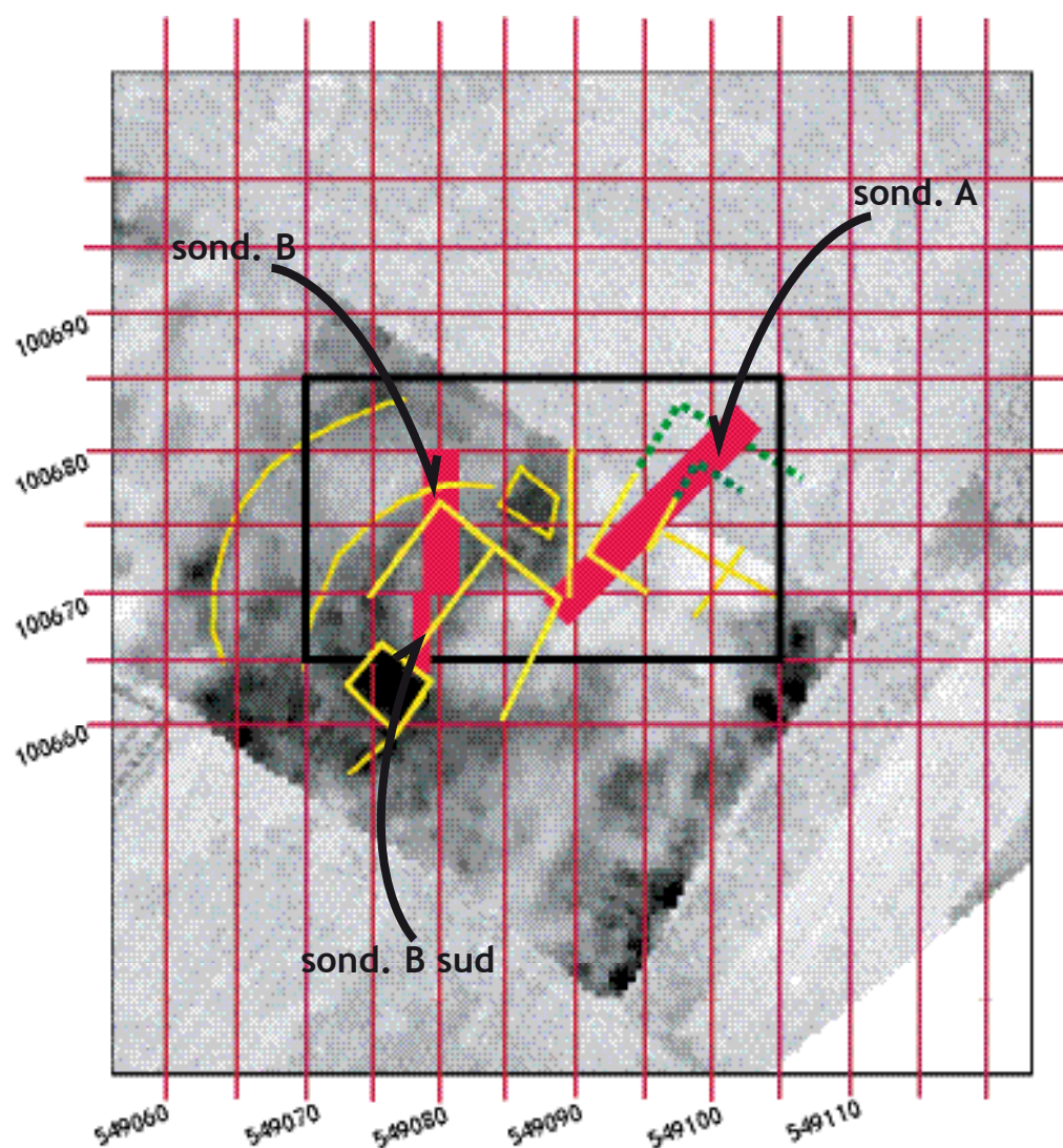
Fig. 27 – Implantation des sondages A (est) et B (ouest) (doc. F. Dugast, 2007).
