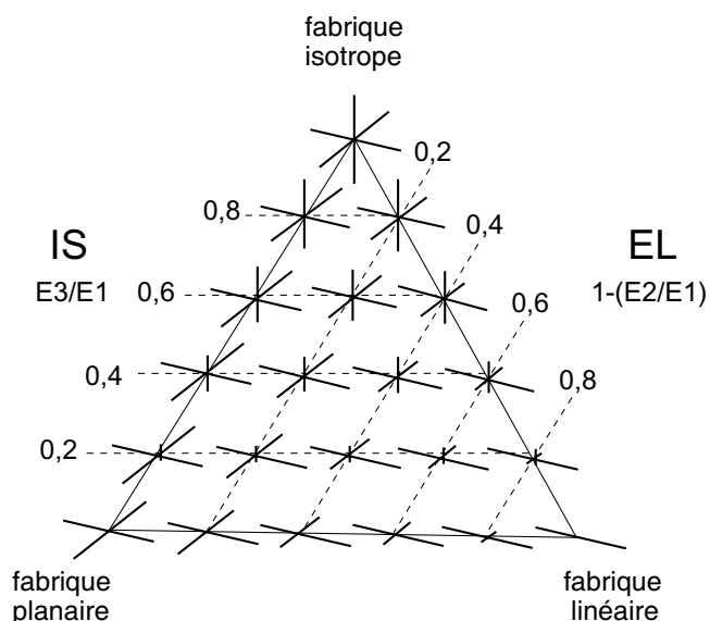
Fig. 6 - Diagramme de Benn
