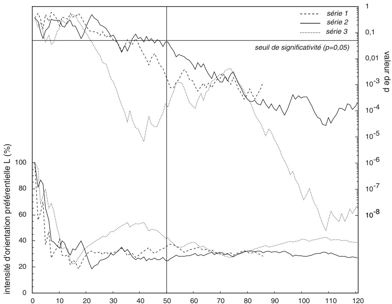
Fig. 2 - Evolution des paramètres L (en haut du diagramme) et p en fonction du nombre de mesures pour trois échantillons différents
