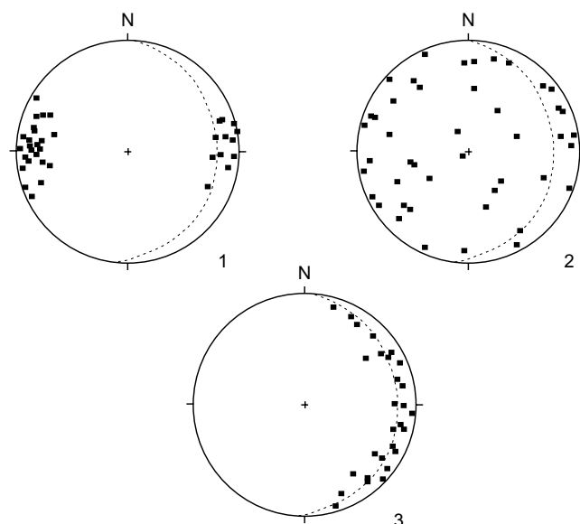
Fig. 4 - Diagrammes de Schmidt. 1 – fabrique linéaire (les points représentatifs des axes sont groupés autour d'une direction), 2 – fabrique isotrope (les points sont dispersés), 3 – fabrique planaire (les points se regroupent sur un plan indiqué par le trait pointillé)
