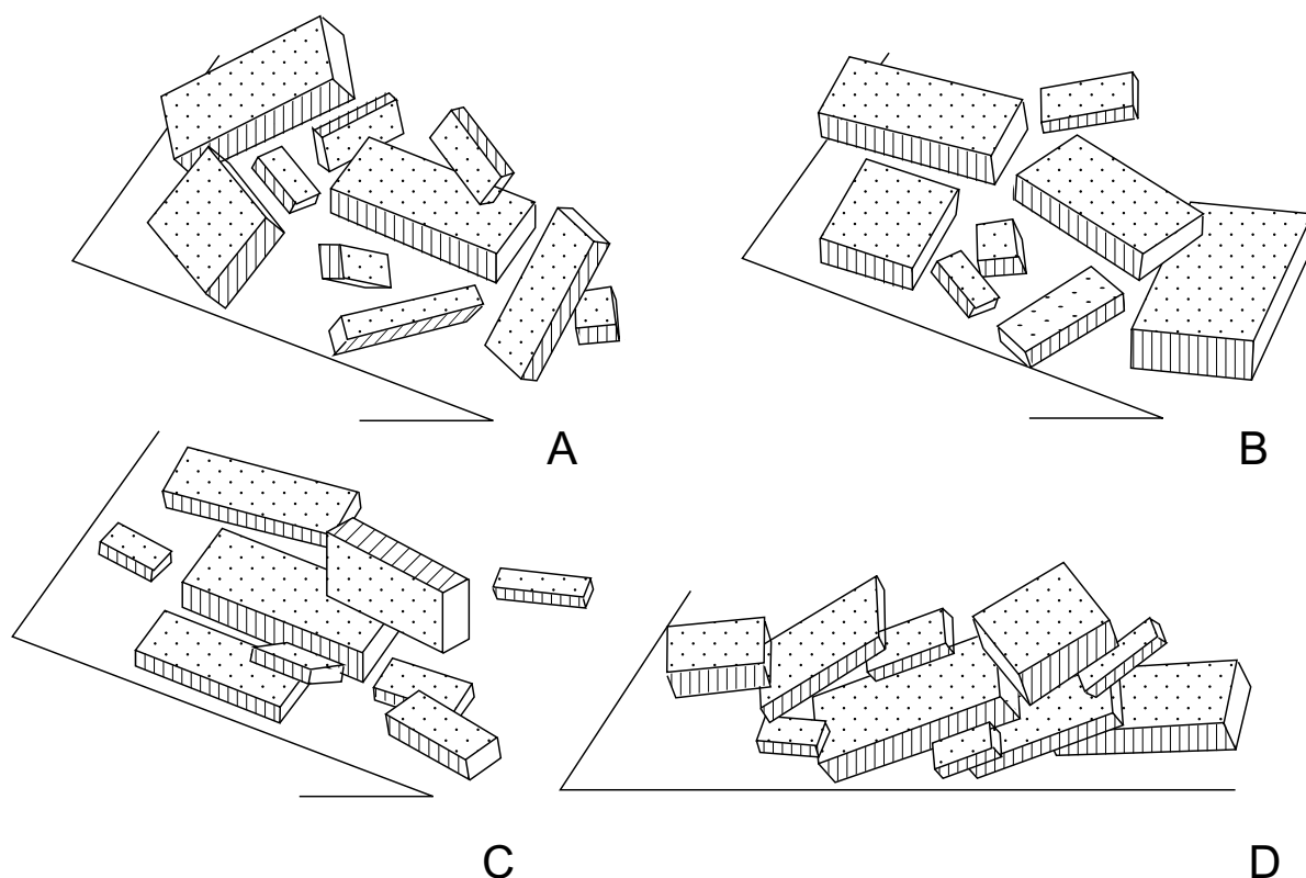
Fig. 1 - Types de fabriques. A – isotrope (désordonnée), B – planaire (à plat sur le plan de stratification), C – linéaire (orientation préférentielle du grand axe des objets), D – imbrication
