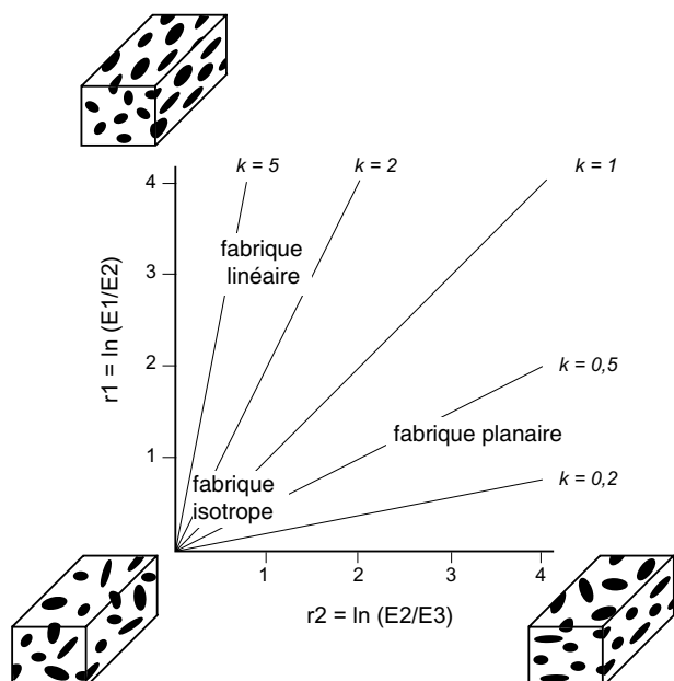
Fig. 5 - Diagramme de Woodcock
