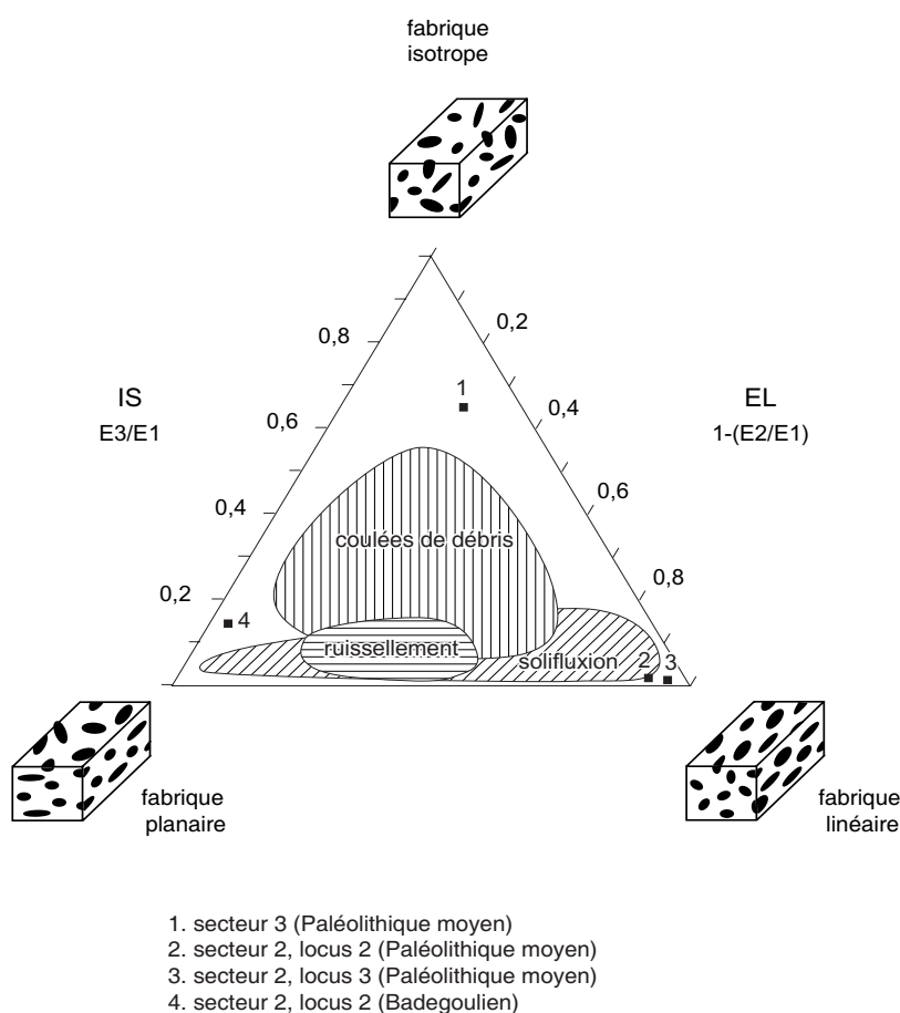
Fig. 12 - Fabriques du site de Croix-de-Canard, diagramme de Benn. Les aires correspondant à différents processus naturels sont indiquées en hachures
