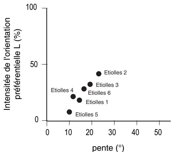
Fig. 10 - Corrélation entre la valeur de la pente et celle du paramètre L (intensité de l'orientation préférentielle) pour le niveau d'occupation D71 du site d'Etiolles. Chaque amas analysé est représenté par un point
