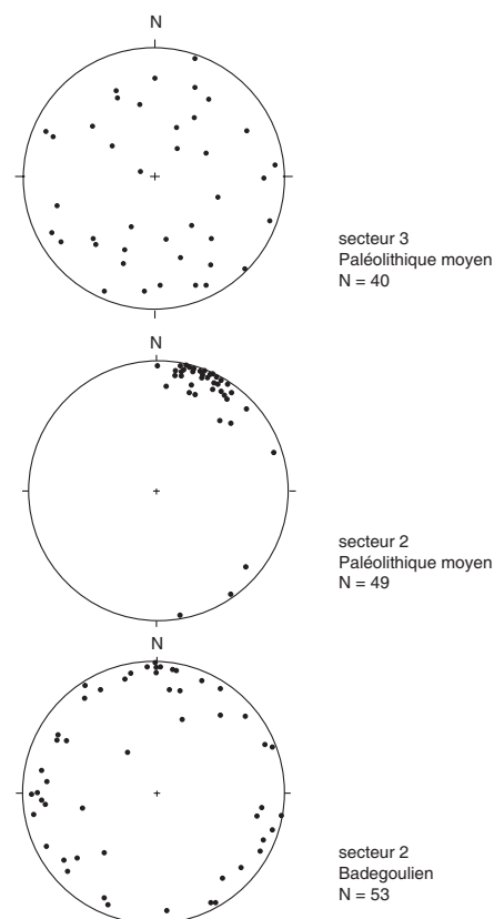
Fig. 11 - Fabriques relevées sur le site de Croix-de-Canard, diagrammes de Schmidt
