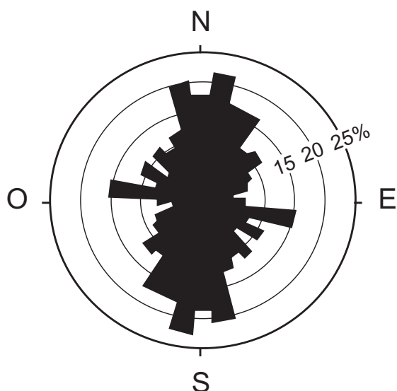
Fig. 3 - Histogramme circulaire des orientations. Exemple provenant d'un niveau moustérien du site de Baume-Vallée (Massif Central), d'après Bertran (1994)
