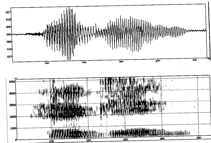
Fig. 9 — Echelle : 100 ms
