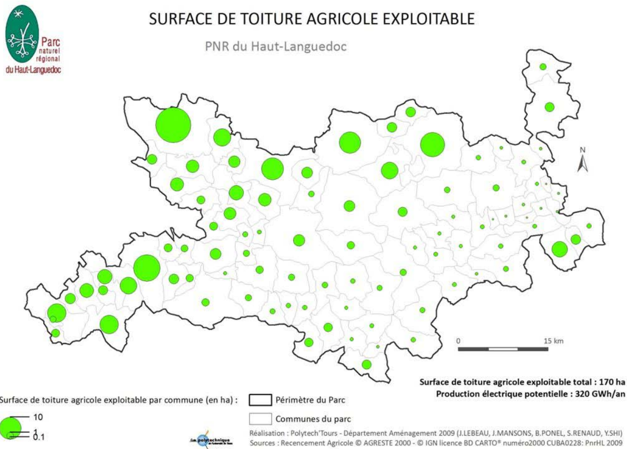
Figure 17 - Localisation et quantification du potentiel en toiture pour les bâtiments agricoles
