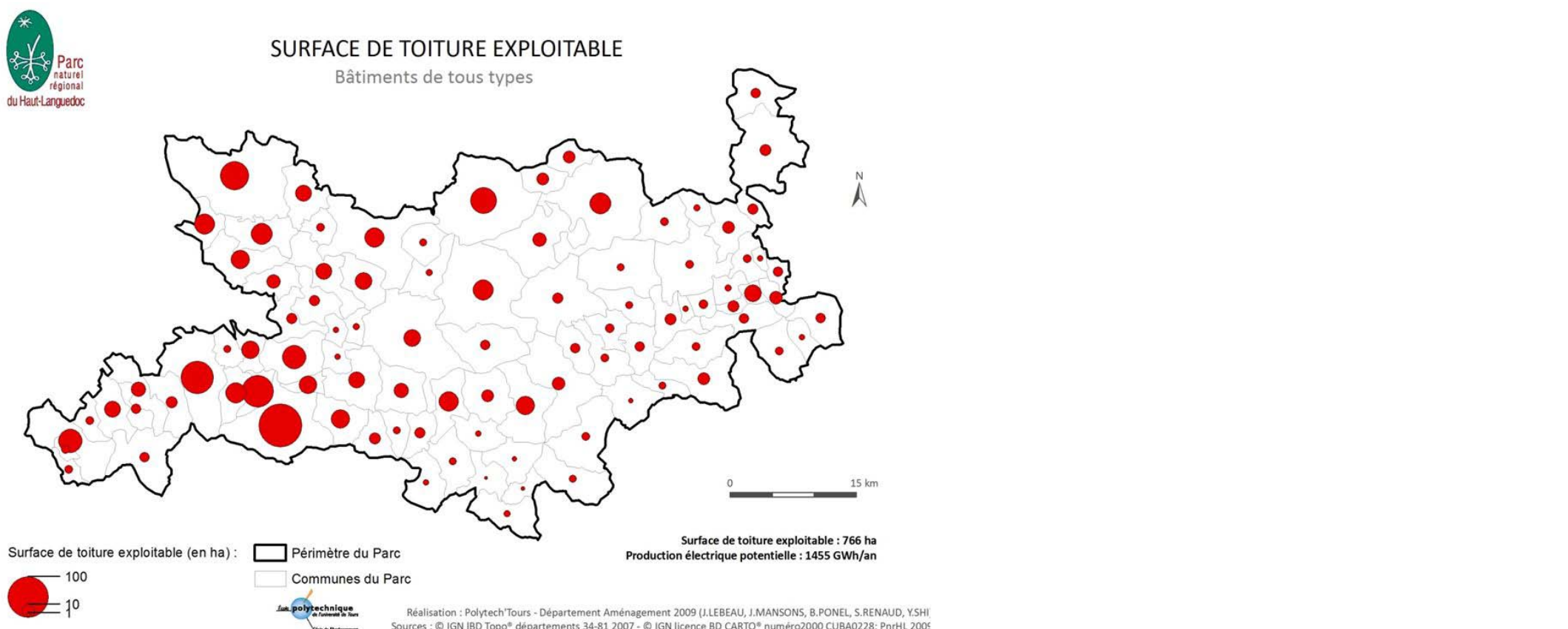
Figure 14 - Localisation et quantification du potentiel en toiture pour tous types de bâtiments (excluant sites inscrits, classés et périmètres de protection)
