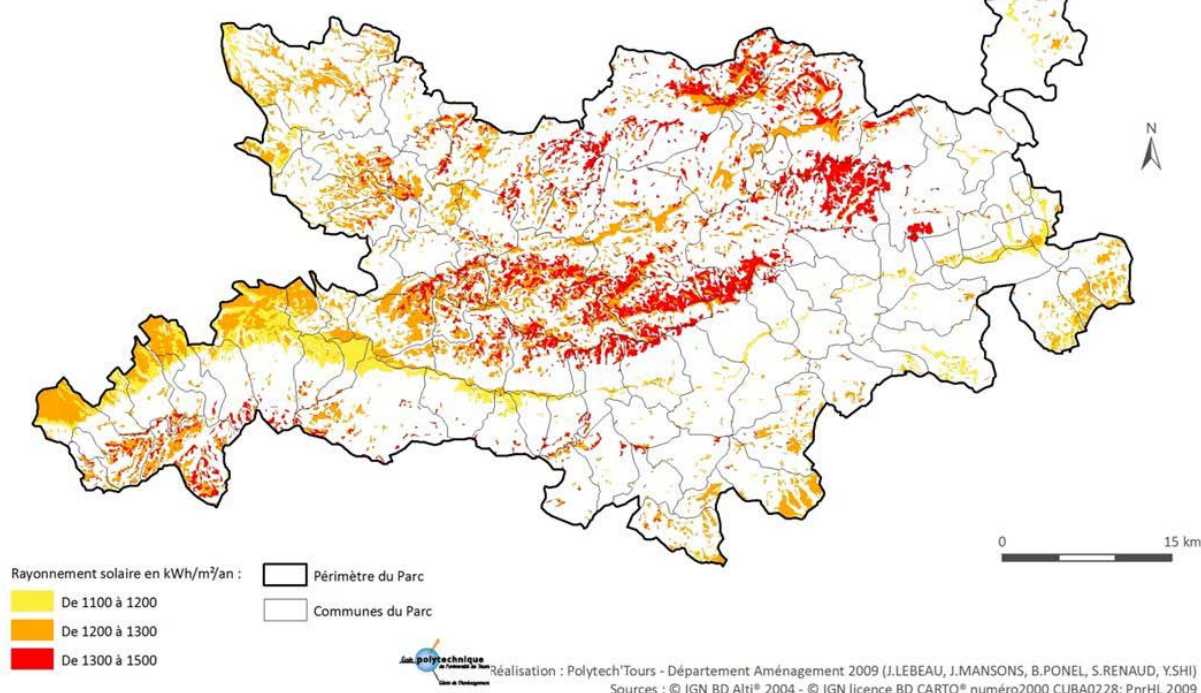
Figure 13 - Zones techniquement exploitables et rayonnement favorable
