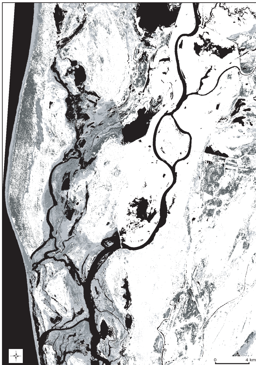
Figure 4 : Sables vifs et processus de salinisation des sols entre 1992 et 2001 (masques à partir de classifications diachroniques non supervisées sur les 3 premiers axes d'ACP des canaux bruts de 1992 et 2001)
