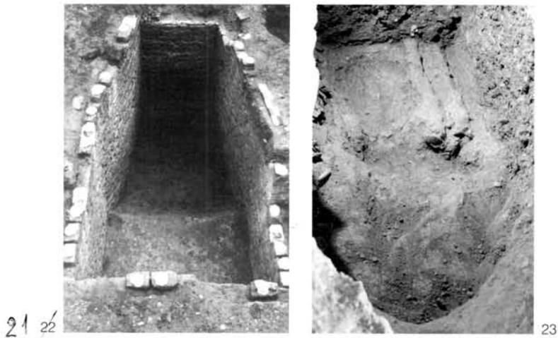
figg. 22-23 – 22. Grand four du Testar del Moli à Paterna, XV e s.a: sagén, b: foyer (cliché J.T.); 23. Four 1424 à 3 banquettes et bassin en arrière du foyer de la C. Crist de la Fé à Paterna, XV e s.? (cliché J.T.).
