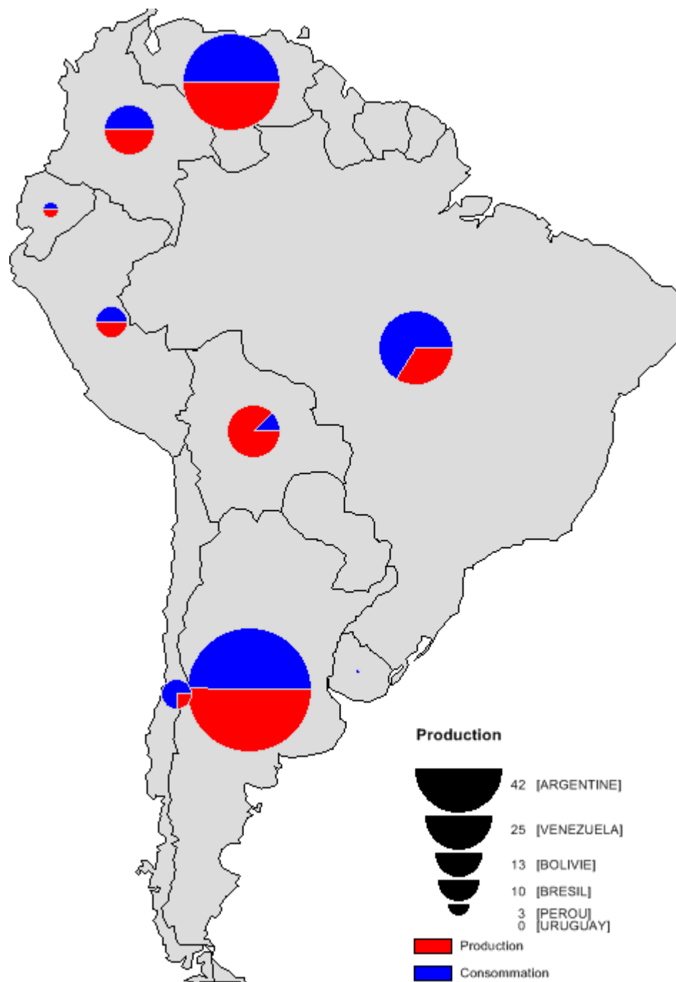
Carte 1 — Proportion entre la production et la consommation de gaz naturel en Amérique du sud, en Mtep :
