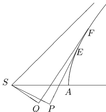
FIG. 1 – L’excès de la tangente sur l’arc d’hyperbole
