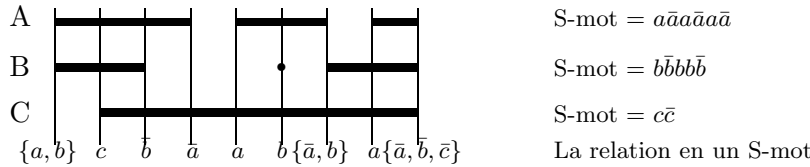
FIG. 1 – Exemple d'une relation ternaire
