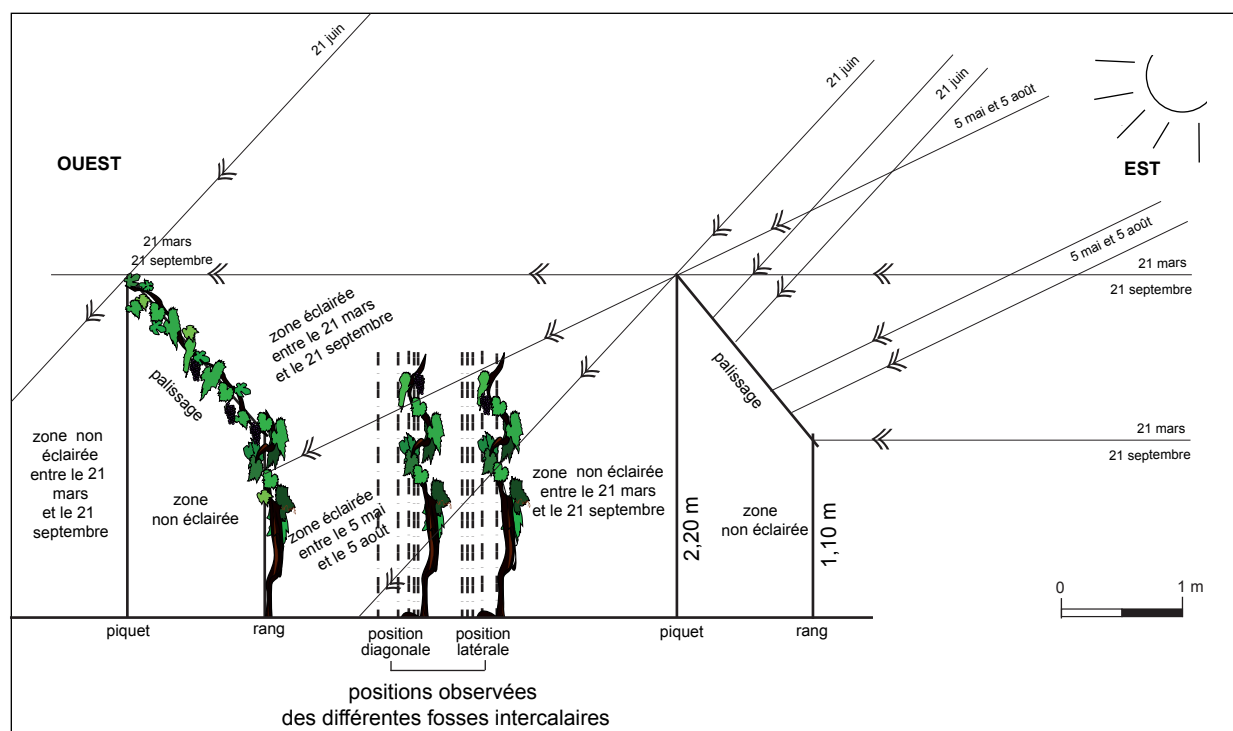
Fig. 29. Modèle d'organisation des pieds de vigne et de leur palissage. Les rangs de piquets sont situés à l'ouest des rangs. Leur distance et l'efficacité énergétique imposent un palissage oblique orienté vers l'est d'environ 40°, ce qui implique une hauteur maximale d'environ 2,20 m pour les piquets. Ce dispositif impose à son tour une zone maximale éclairée entre les rangs, le matin, sur la moitié ouest de l'inter-rang. C'est précisément là que l'on a observé l'implantation des fosses intercalaires.
