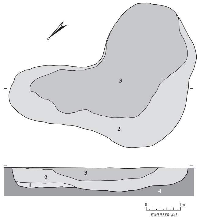
Fig. 4. Relevé de la fosse d'extraction n° 1.
