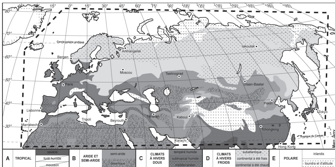
1. Carte climatique de l'Eurasie (selon Köppen 1936) Les tirets délimitent l'espace couvert par les espèces et les stations météorologiques de référence (D.A.O. : Marc Jarry) / 1. Eurasian climatic map (from Köppen 1936) Dotted line delineates the space covered by referential species and weather stations
