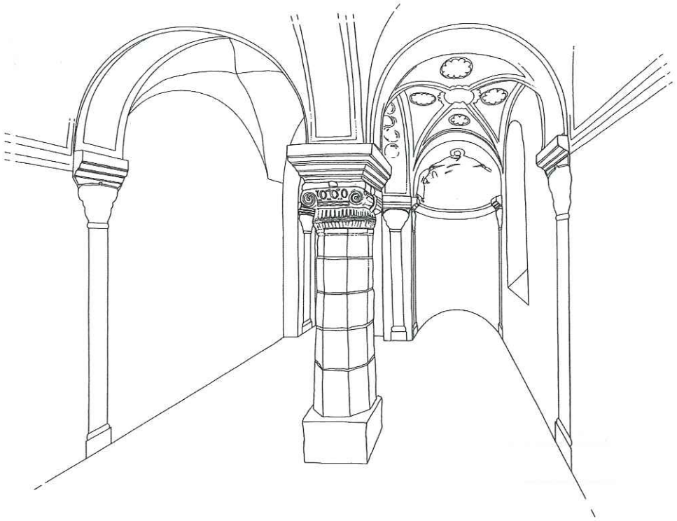
Fig. 5. Vue restituée de l'oratoire Saint-Laurent (dessin G. Fèvre, CEM, 2000)
