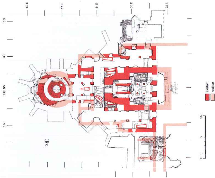
Fig. 3B. Plan de l'état carolingien de la crypte (CEM, 2000)
