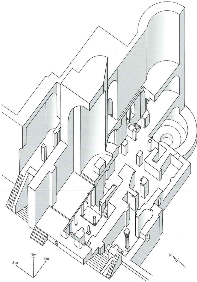
Fig. 1. Auxerre, crypte de Saint-Germain, restitution axonométrique (dessin G. Fèvre, CEM, 2000)
