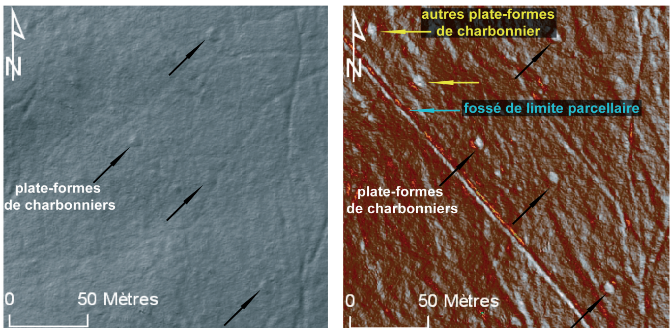
Fig. 5. Plates-formes de charbonniers et fossé limite de parcelle vus suivant un traitement ombrage 315° 45° et suivant un traitement pente (zone de Besançon) (SIG & DAO programme LIEPPEC © MSHE C. N. Ledoux, C. Fruchart)
