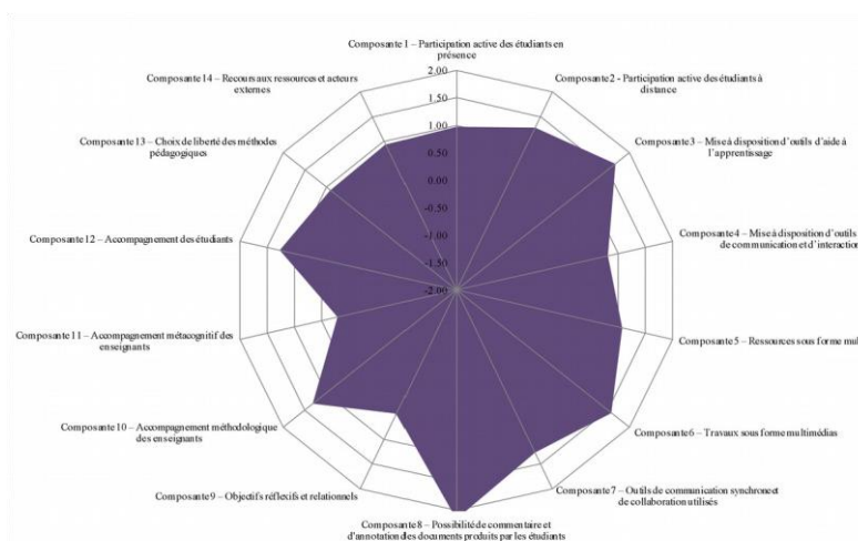
Graphique 6. Scores factoriels du type 6 selon les 14 composantes
