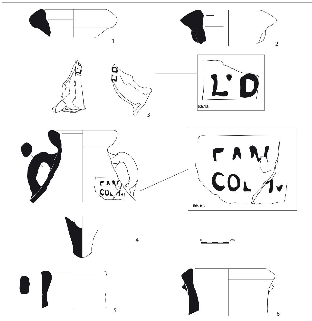
Fig. 18. Les amphores. Période 1 et 2 (éch. 1/3) (S. Mouton-Venault, DAO Y. Amrane).
